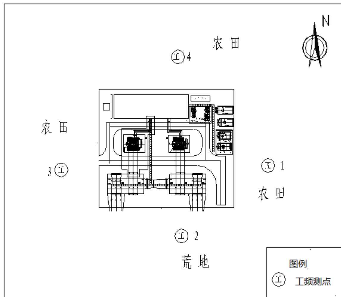
附图 4 110kV 西湖变电站（类比站）监测点位示意图
