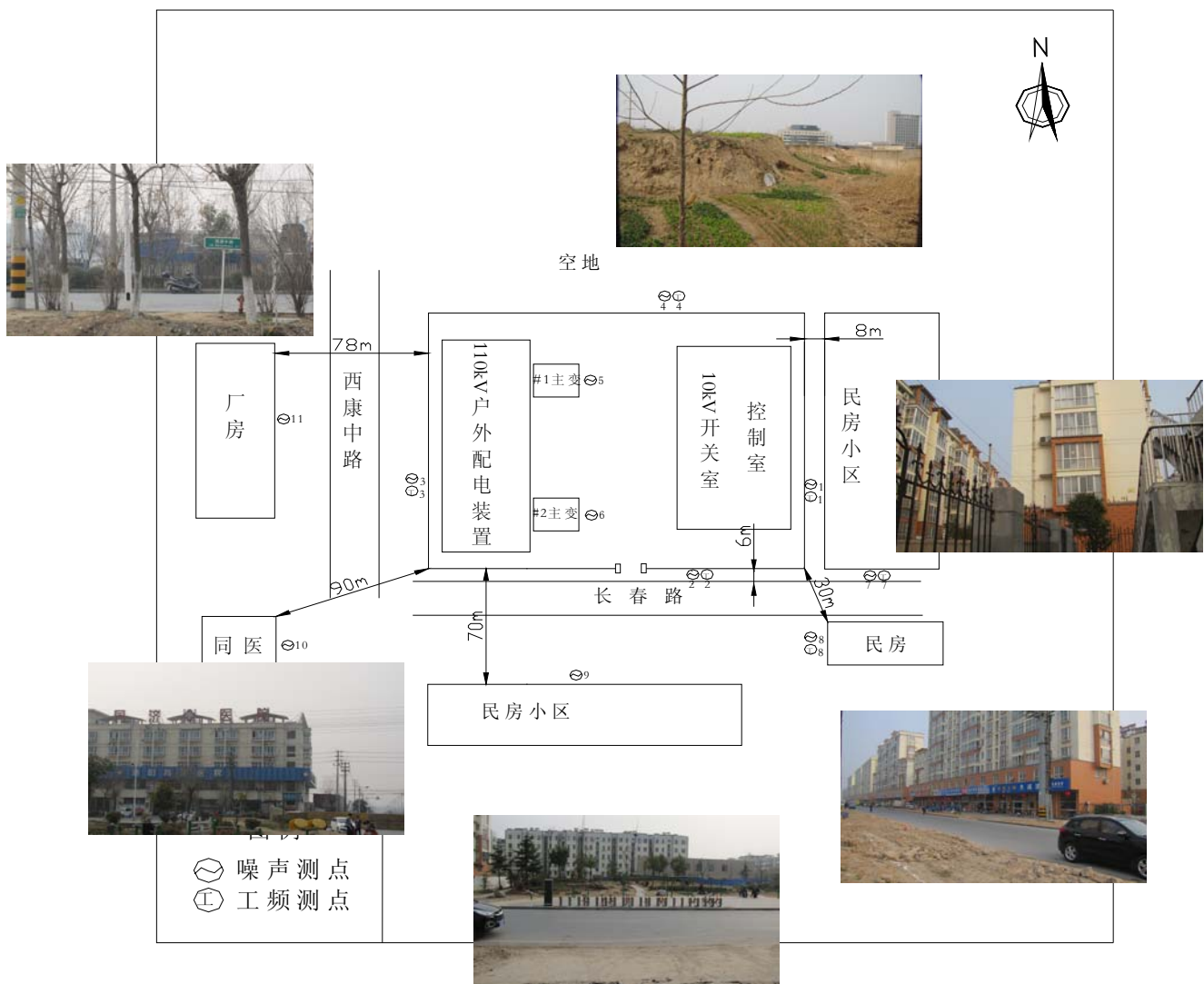
附图2 110kV 郑庄变电站监测点位及周围环境示意图
