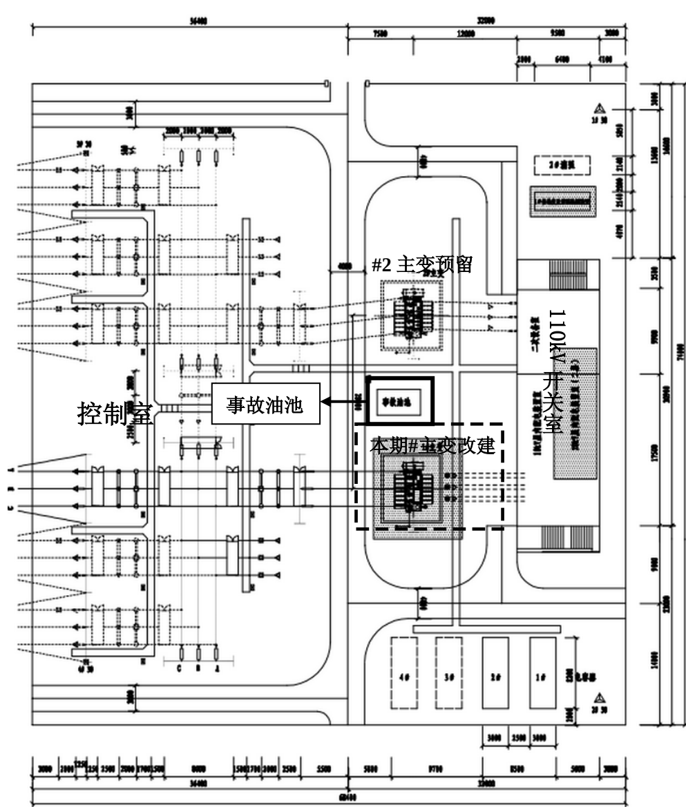
附图 3 110kV 杜村变平面布置示意图
