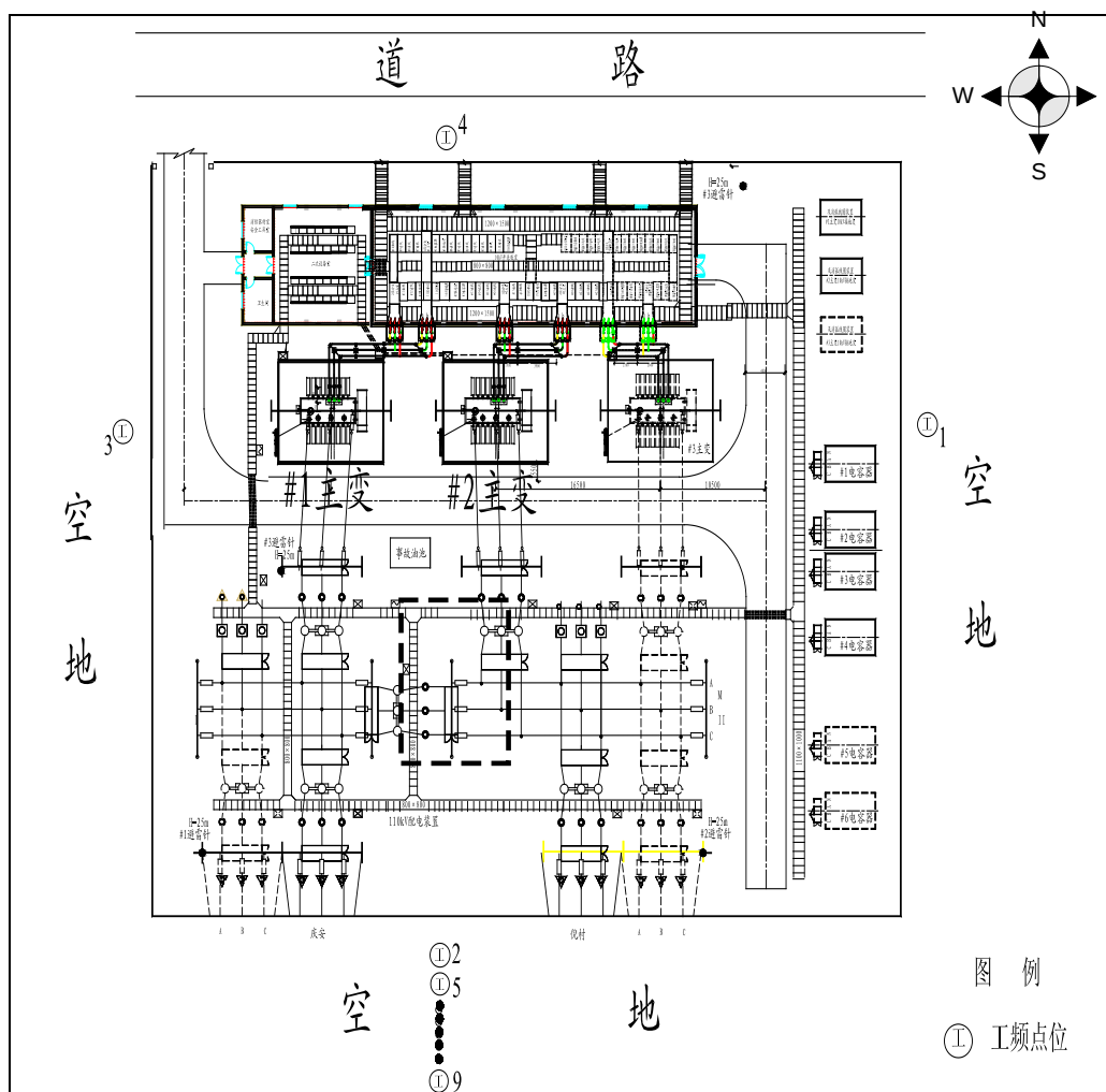
附图 4 110kV 联群变电站（类比站）监测点位示意图
