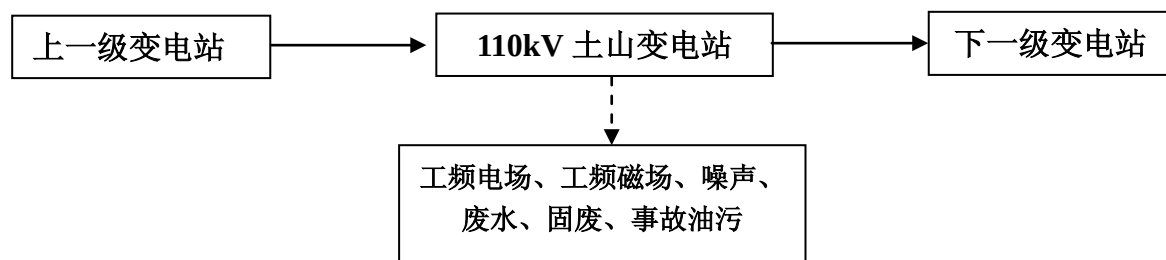
图 2 110kV 土山变电站工程工艺流程及产污环节示意图
