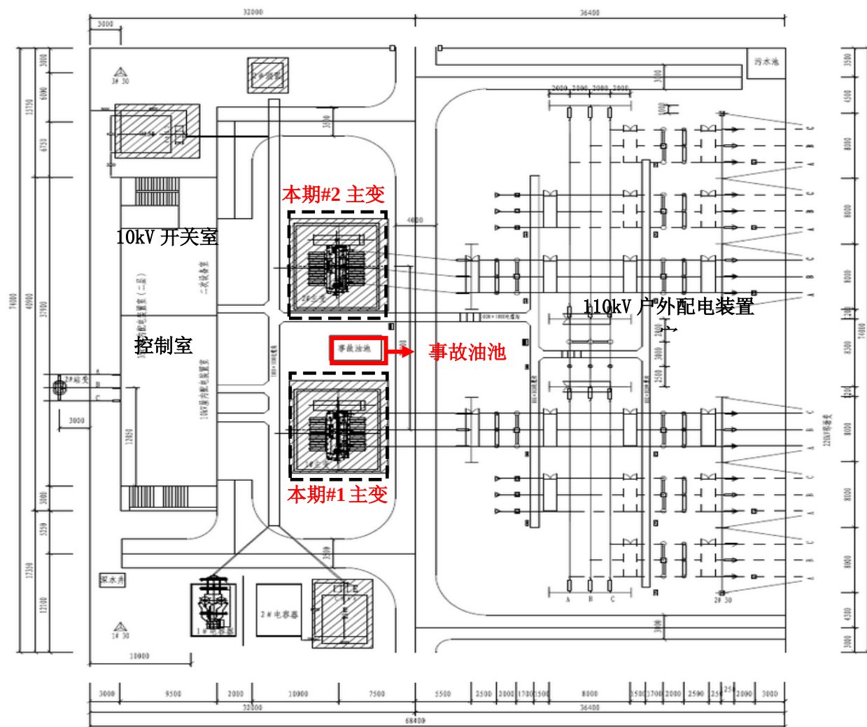
附图 3 110kV 土山变电站平面布置图
