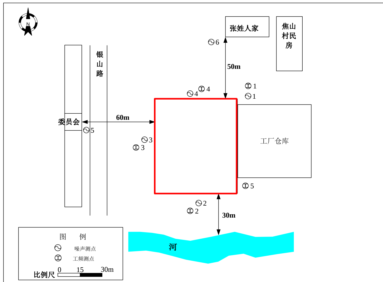
附图 2 110kV 焦山变电站检测点位及周围环境示意图
