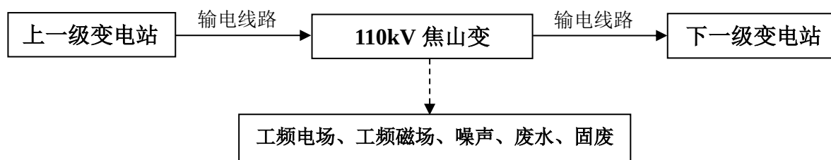
图 1 110kV 焦山变#2 主变增容工程工艺流程及产污环节示意图
