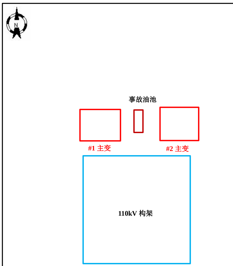
附图 3 110kV 焦山变电站总平面布置图
