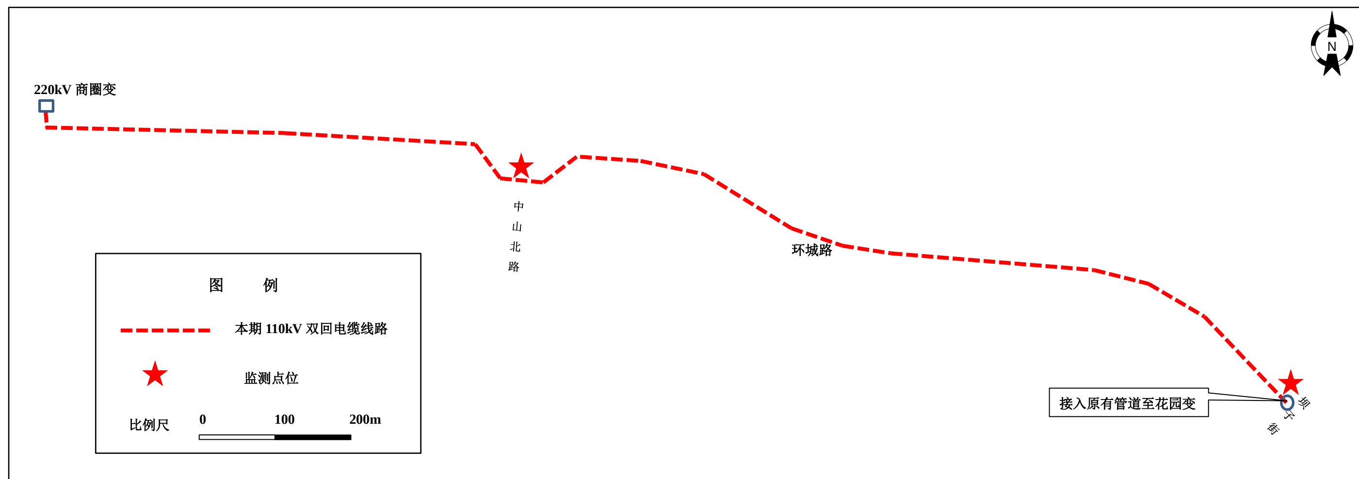
附图 2 徐州 110kV 秦洪变至花园变 \pi 入商圈变线路工程线路路径示意图 (a)
