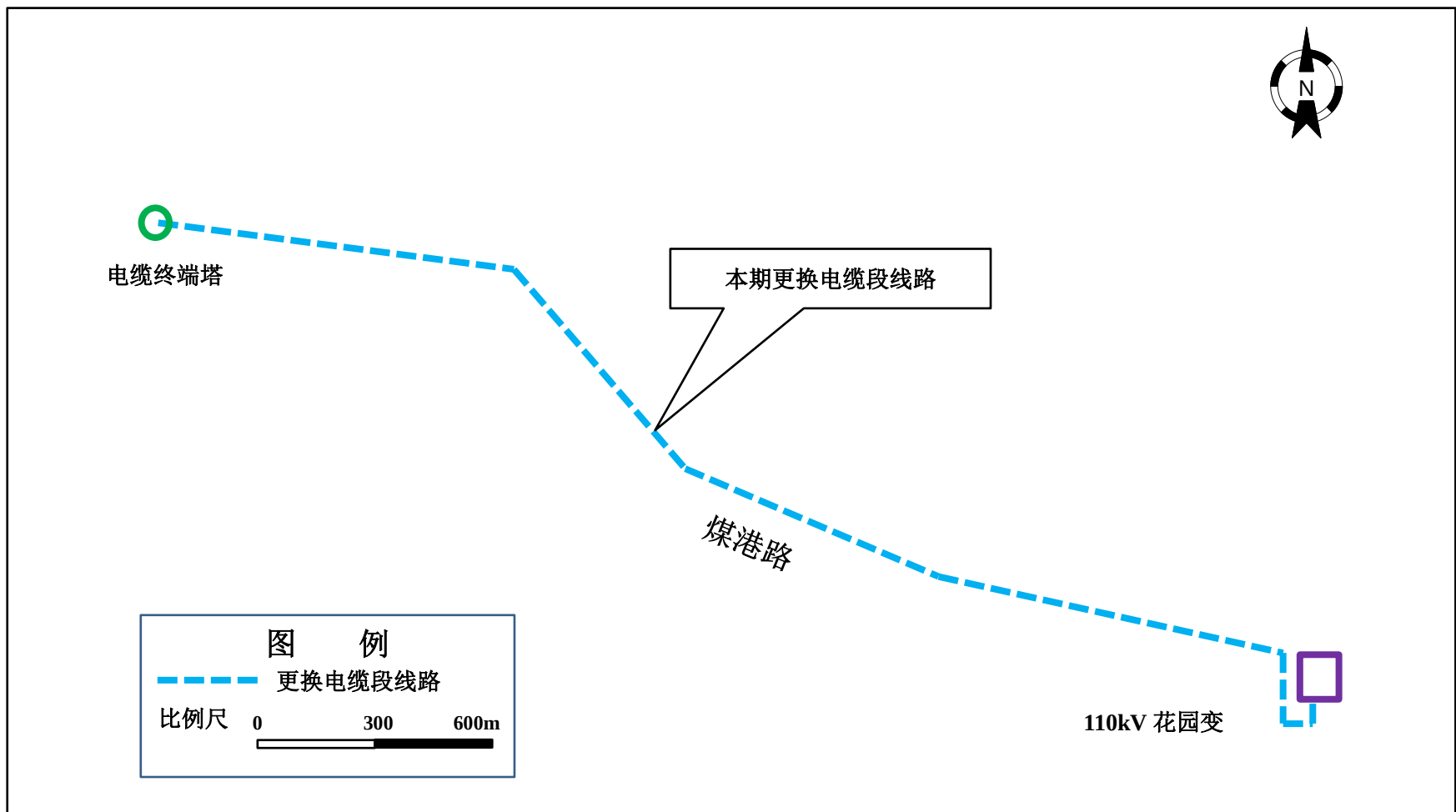
附图 2 徐州 110kV 秦洪变至花园变 \pi 入商圈变线路工程线路路径示意图 (b)
