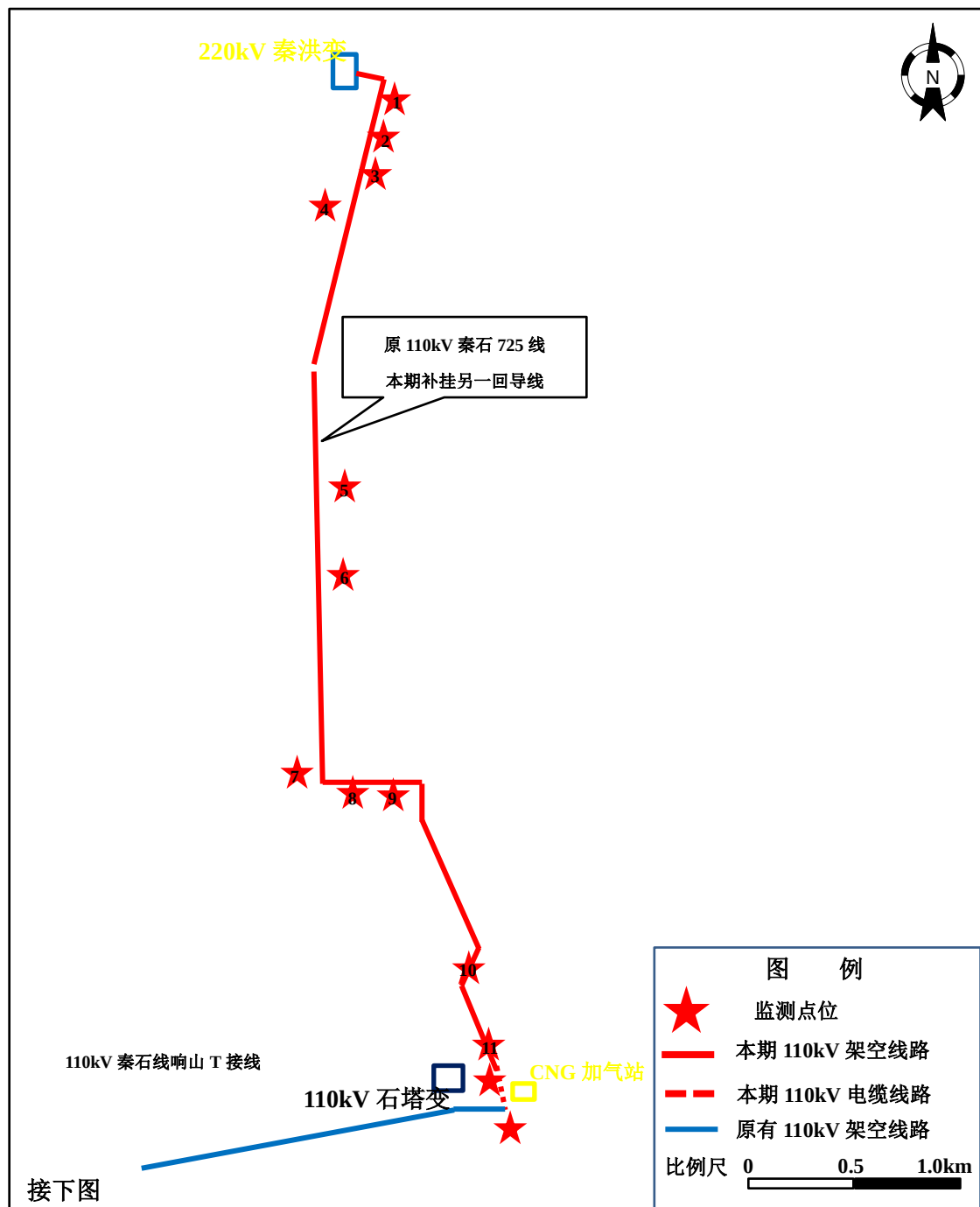
附图 2 110kV 线路路径及监测点位示意图 (a)
