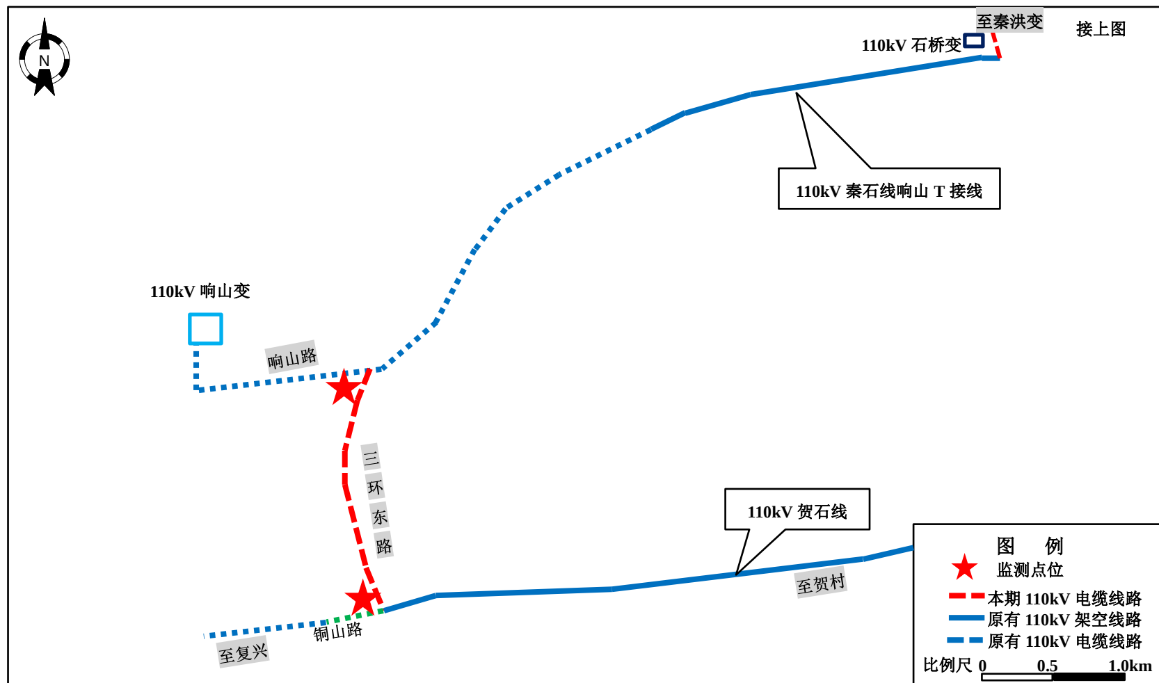
附图 2 110kV 线路路径及监测点位示意图 (b)
