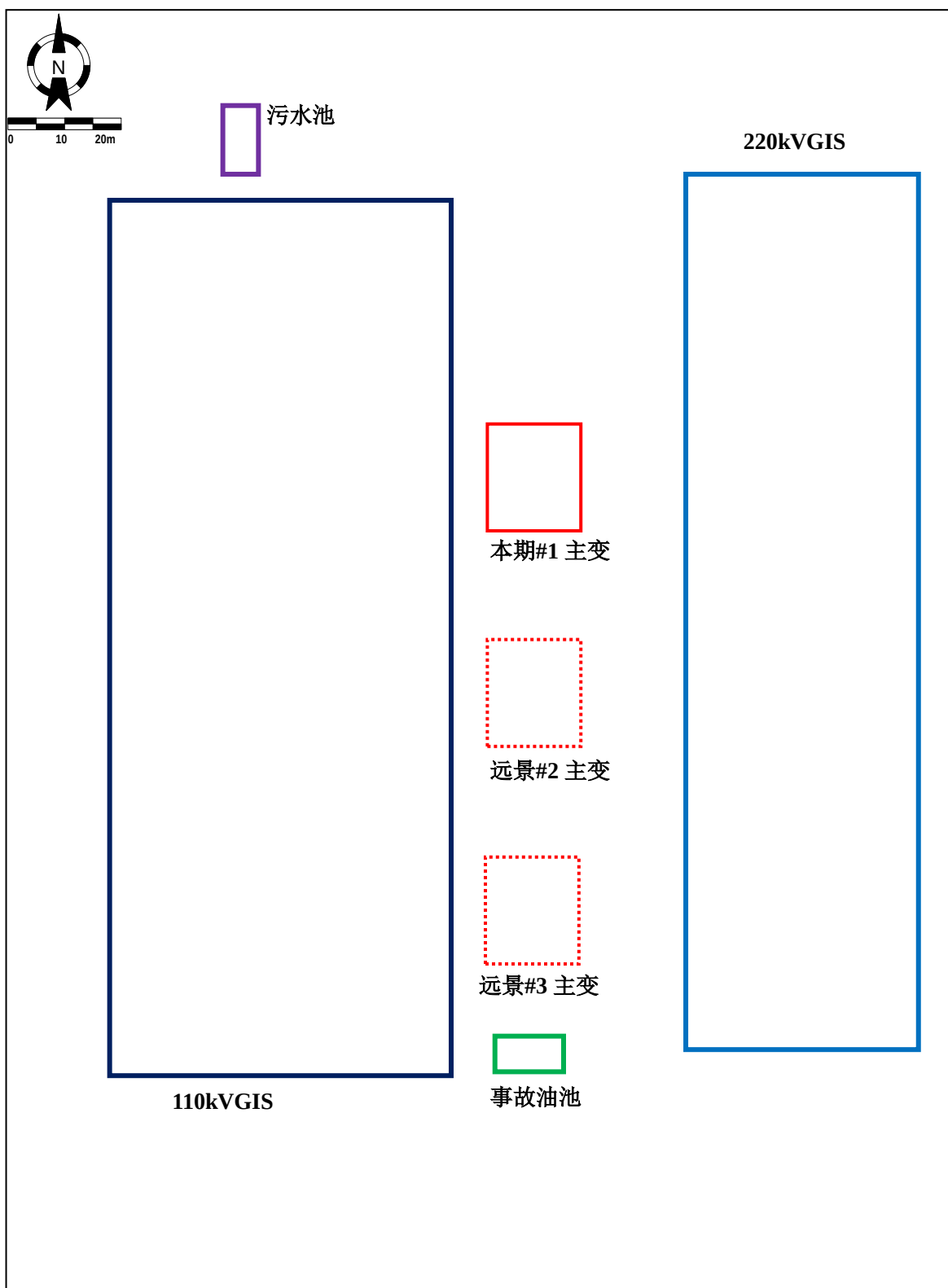
附图 3 220kV 马陵山变电站平面布置图
