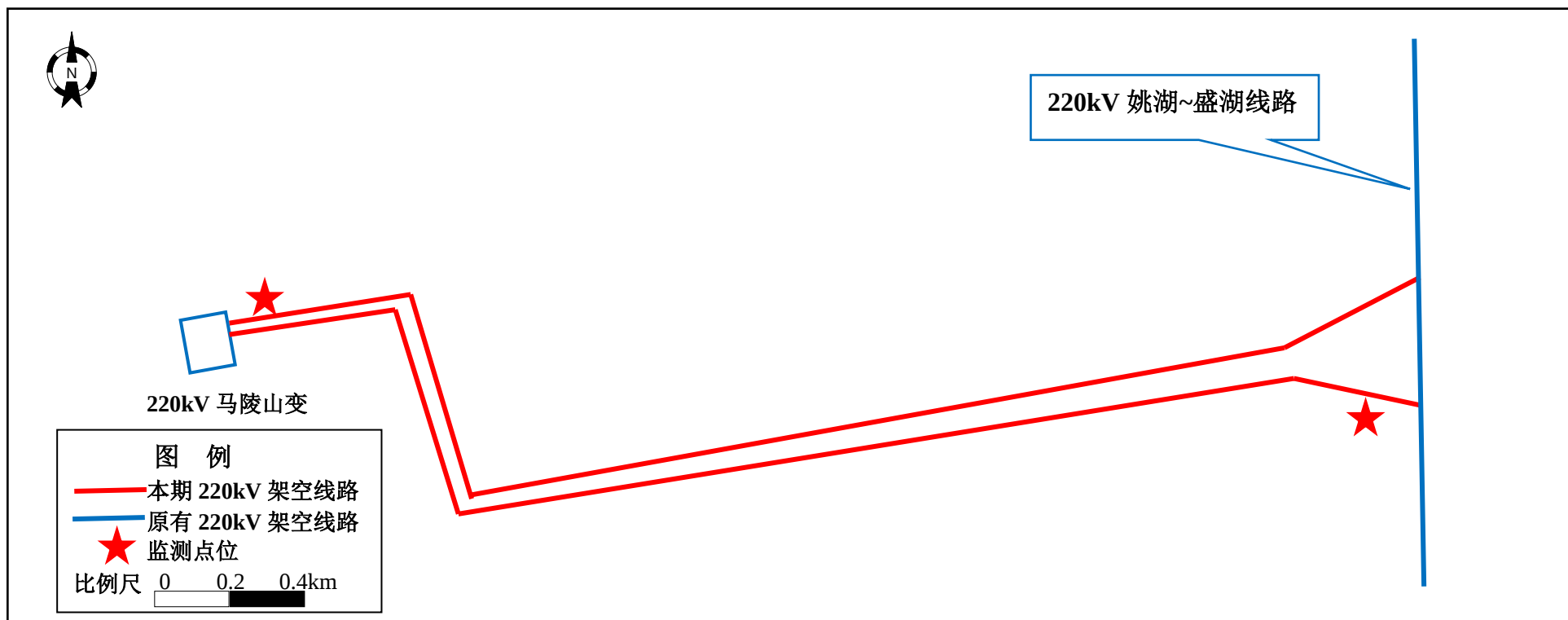
附图 4 220kV 马陵山输变电工程配套线路路径及检测点位示意图
