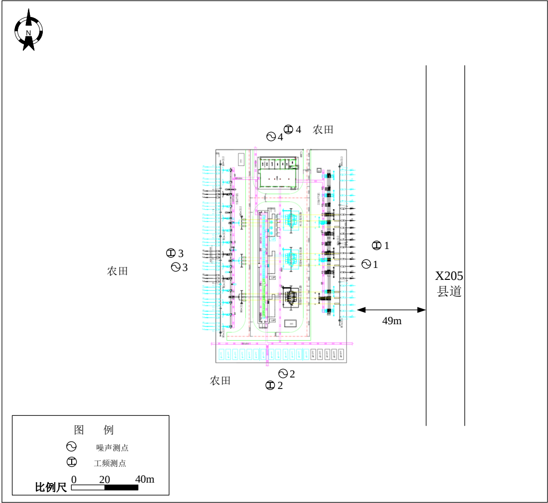
附图 2 220kV 马陵山变电站拟建址周围监测点位及环境示意图
