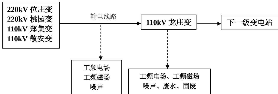
图 1 110kV 输变电工程工艺流程及产污环节示意图
