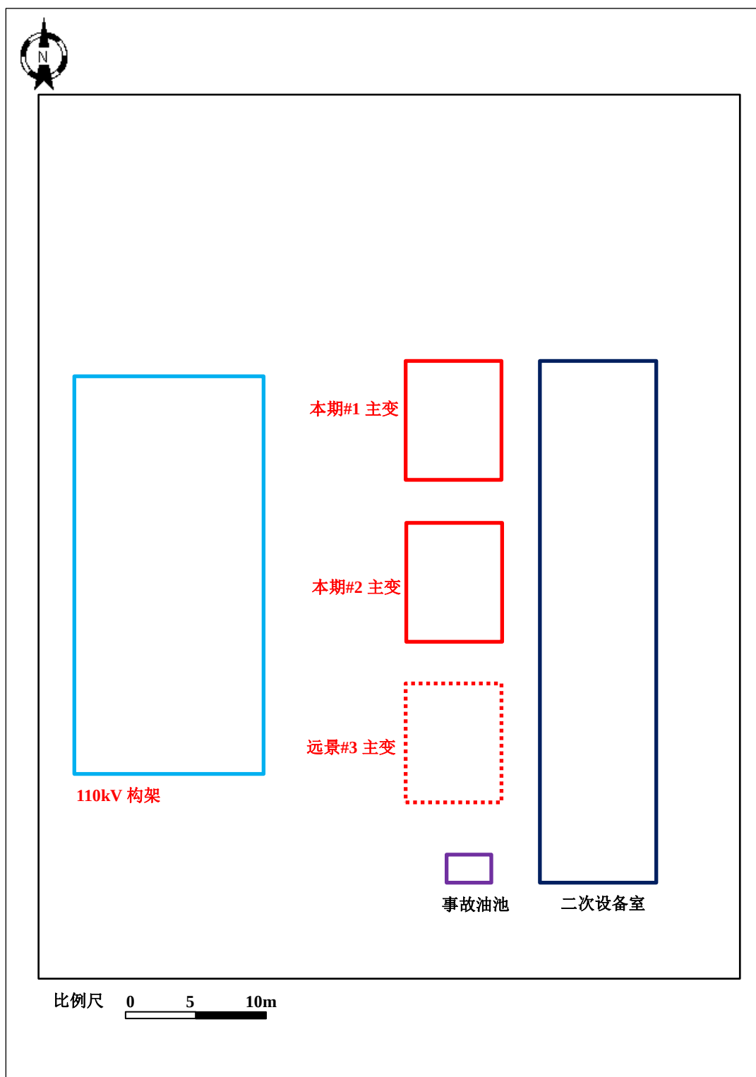
附图 3 110kV 新星（桥上）变总平面布置示意图
