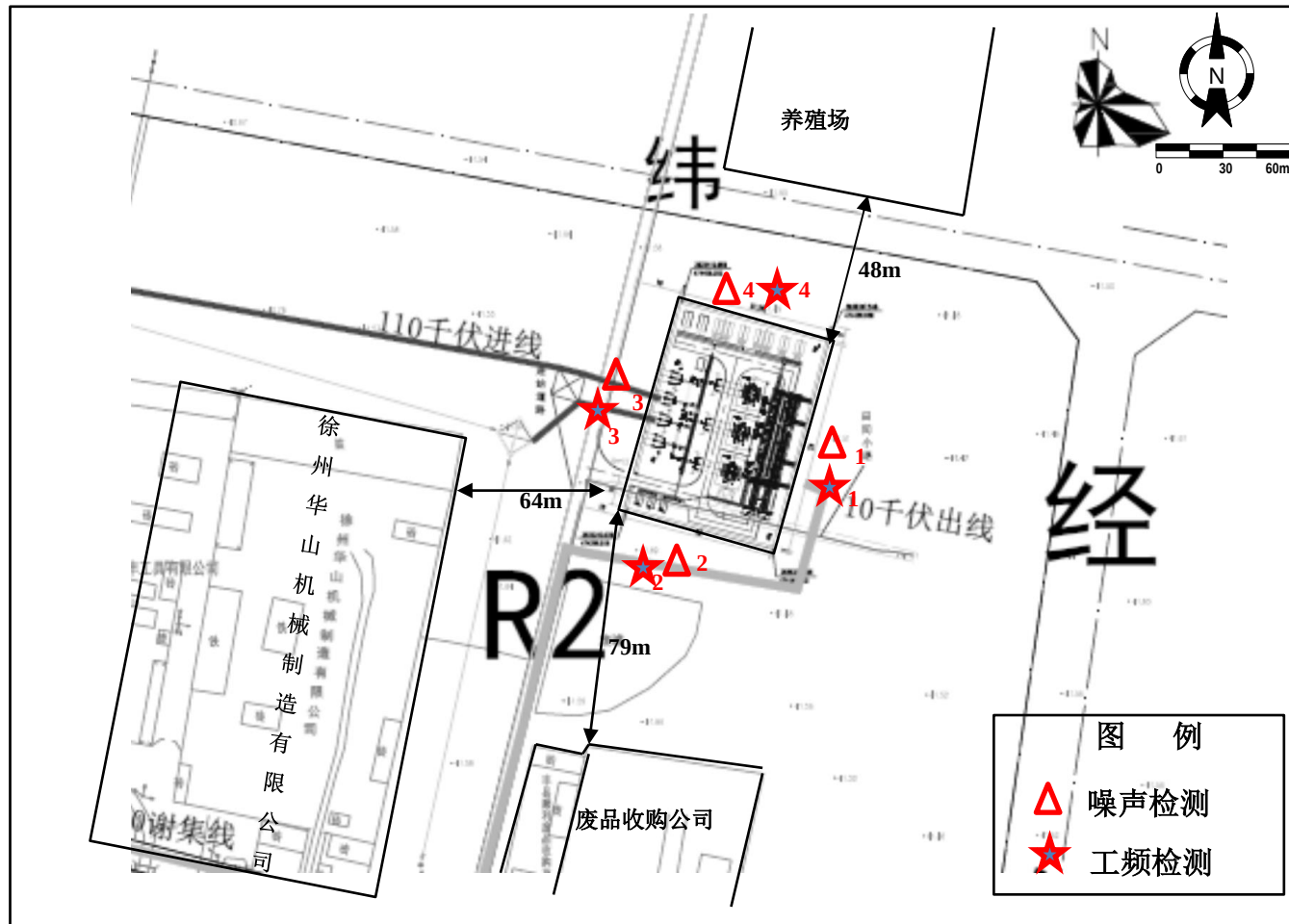
附图2 套楼 110kV 变电站拟建址周围监测点位及环境示意图
