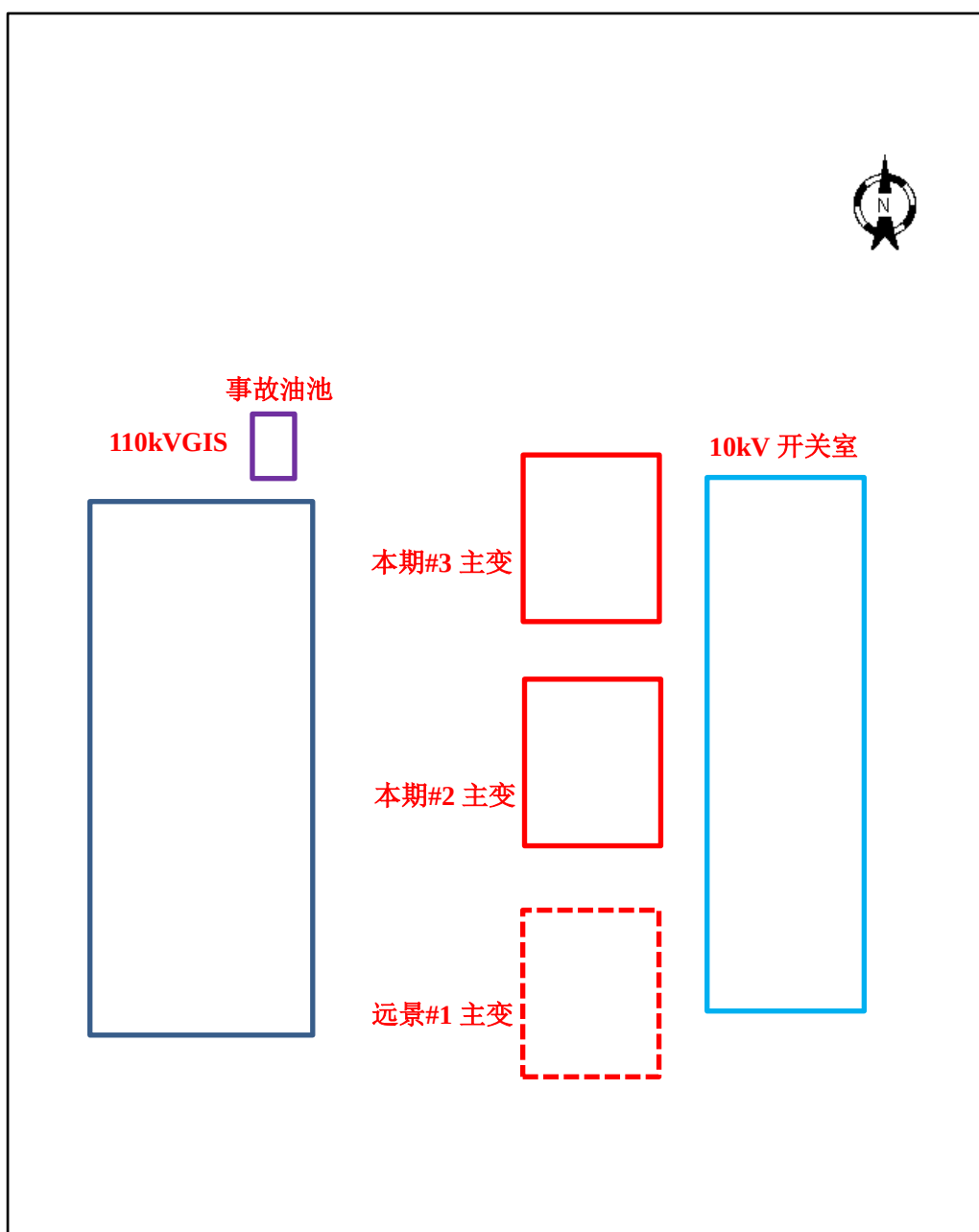
附图3 套楼 110kV 变电站平面布置图
