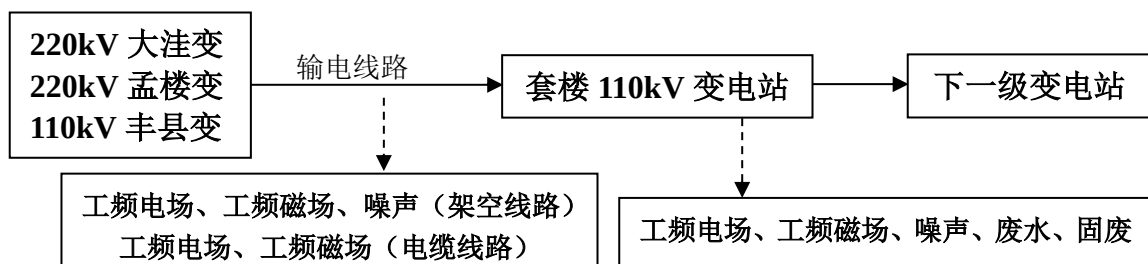
图 1 110kV 输变电工程工艺流程及产污环节示意图
