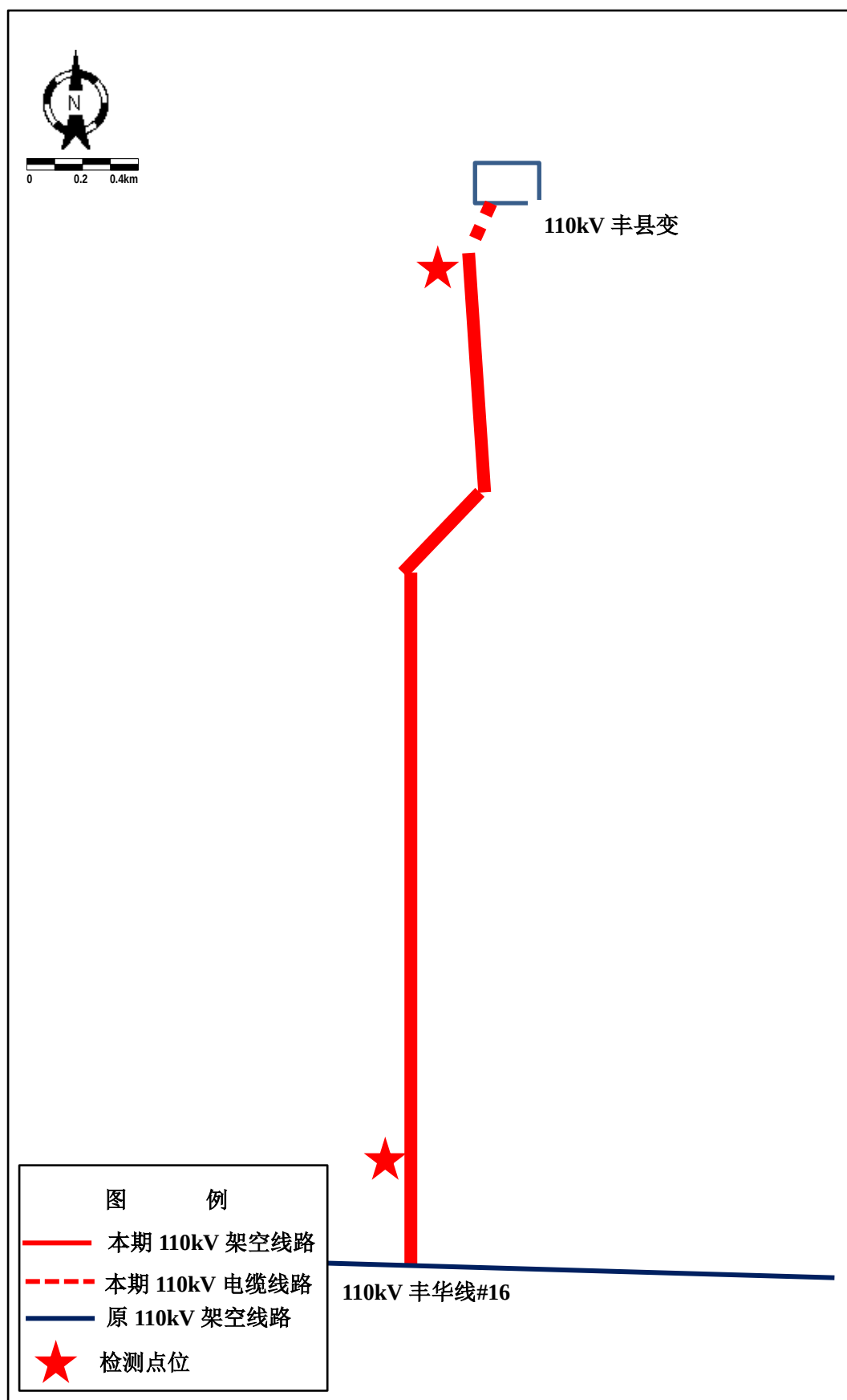
附图 6 110kV 丰华线#1~#16 线路改造工程线路路径及检测点位示意图
