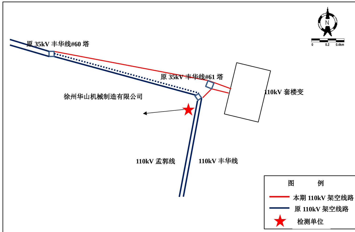
附图 4 110kV 丰华线开断环入套楼变线路工程线路路径及检测点位示意图
