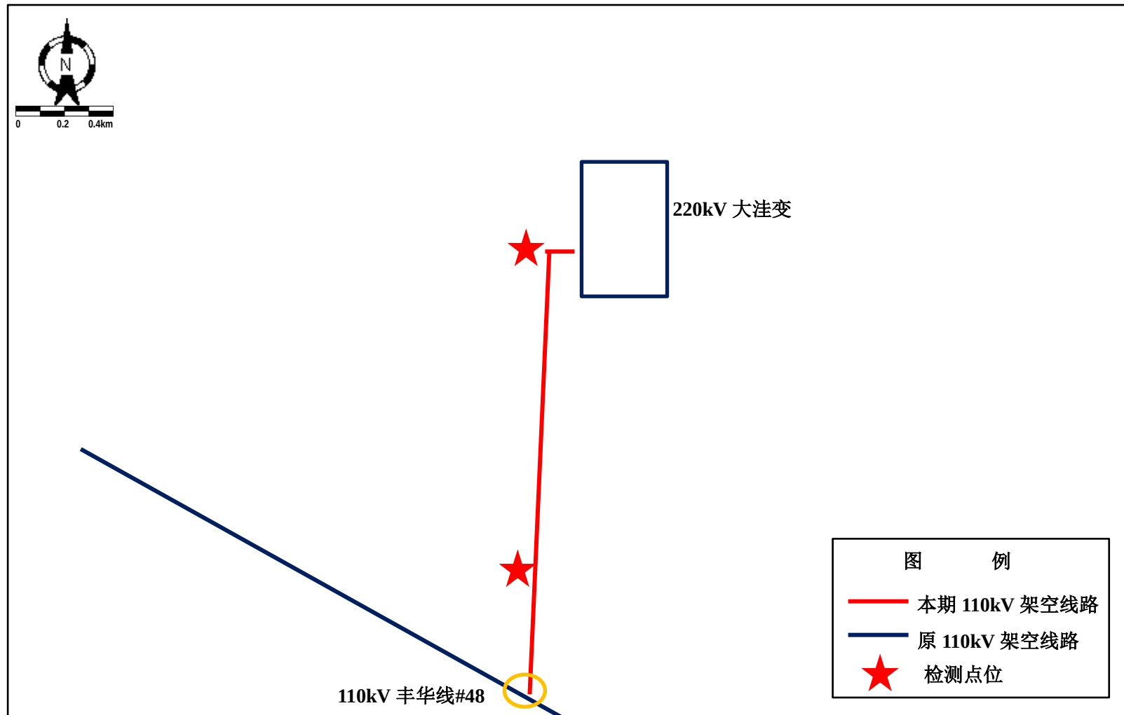
附图 5 110kV 丰华线开断环入大洼变线路工程线路路径及检测点位示意图
