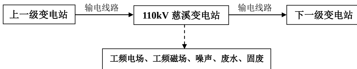
图 1 沭阳 110kV 慈溪变电站扩建#1 主变工程工艺流程及产污环节示意图
