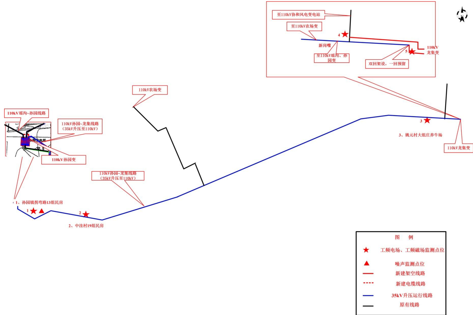
附图4 110kV 龙集变电站配套 110kV 线路路径及监测点位示意图
