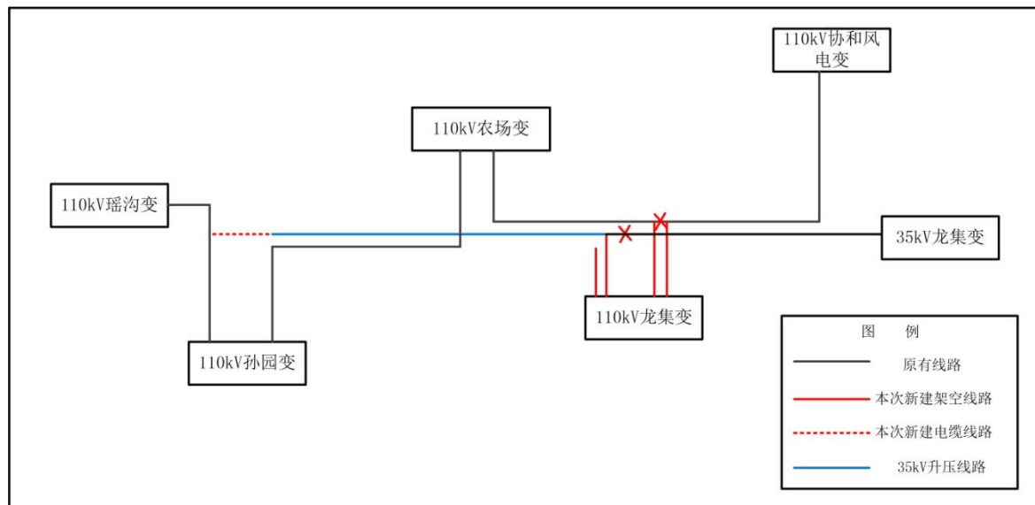
图 1 本工程接线示意图
