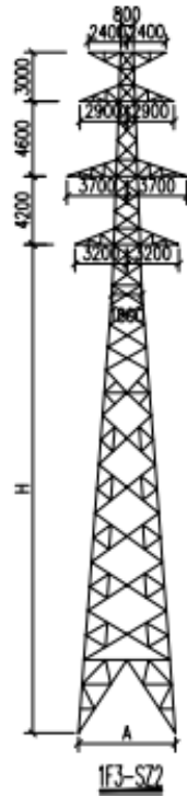
协和风电变至农场变 \pi 入龙集变电站 110kV 线路工程
