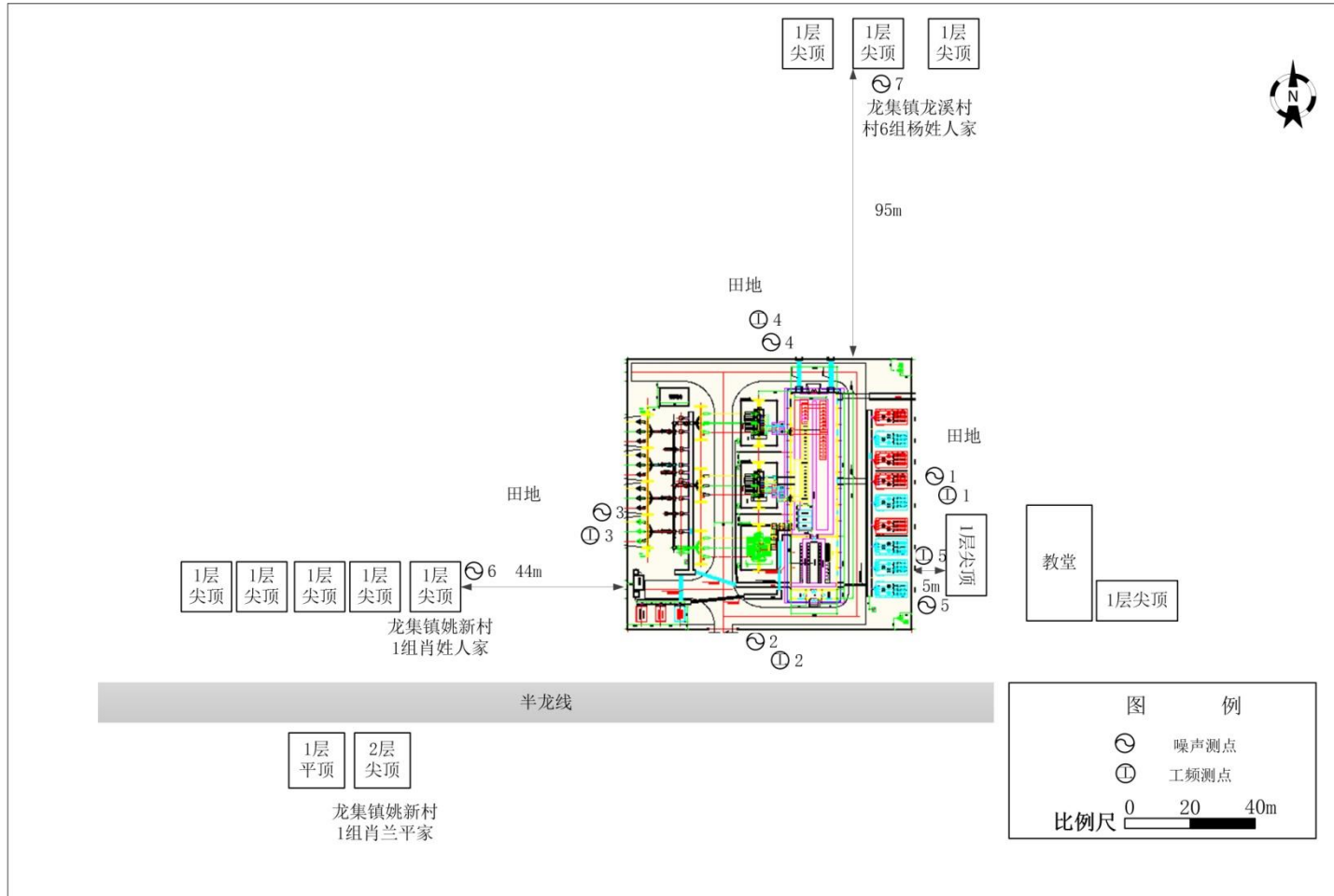
附图 2 110kV 龙集变电站拟建址周围监测点位及环境示意图
