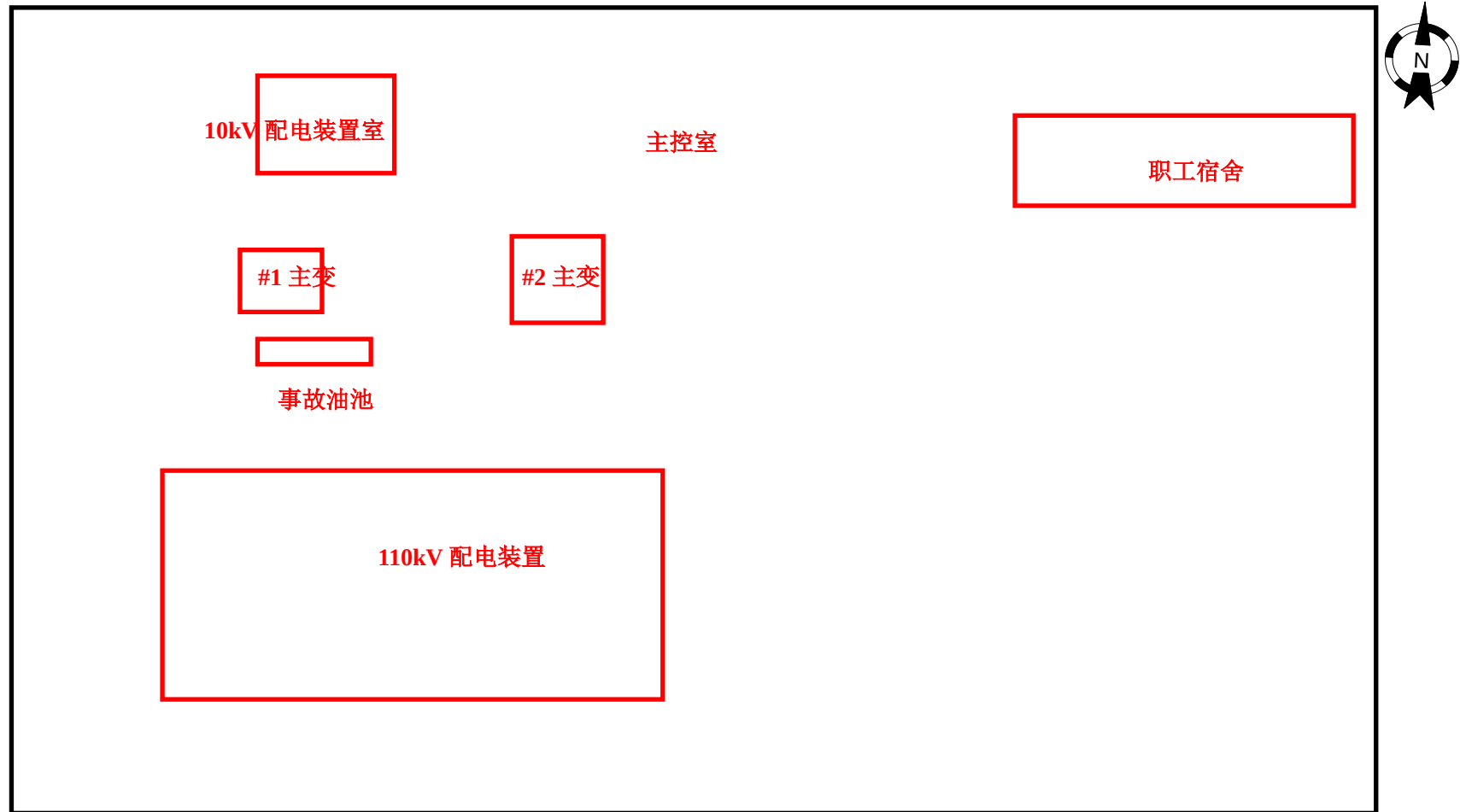
附图 3 110kV 泗洪变电站总平面布置图
