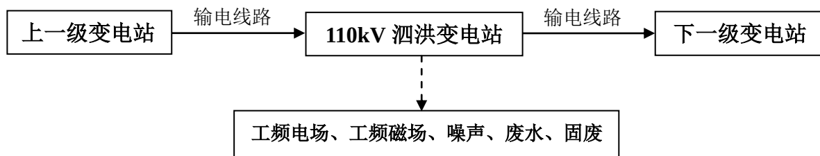
图 1 泗洪 110kV 泗洪变电站主变增容工程工艺流程及产污环节示意图
