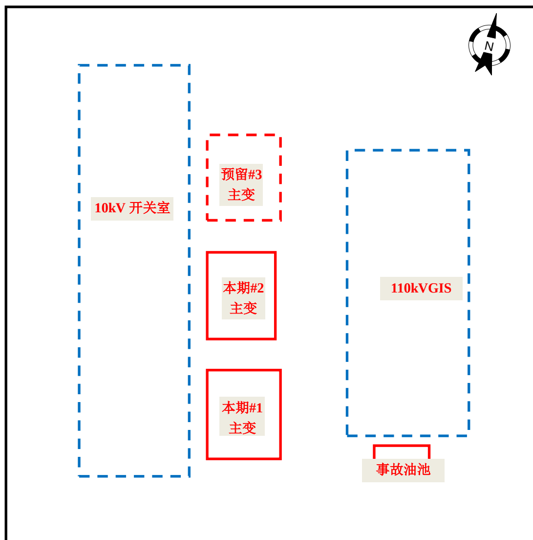
附图3 110kV 爱园变电站总平面布置示意图
