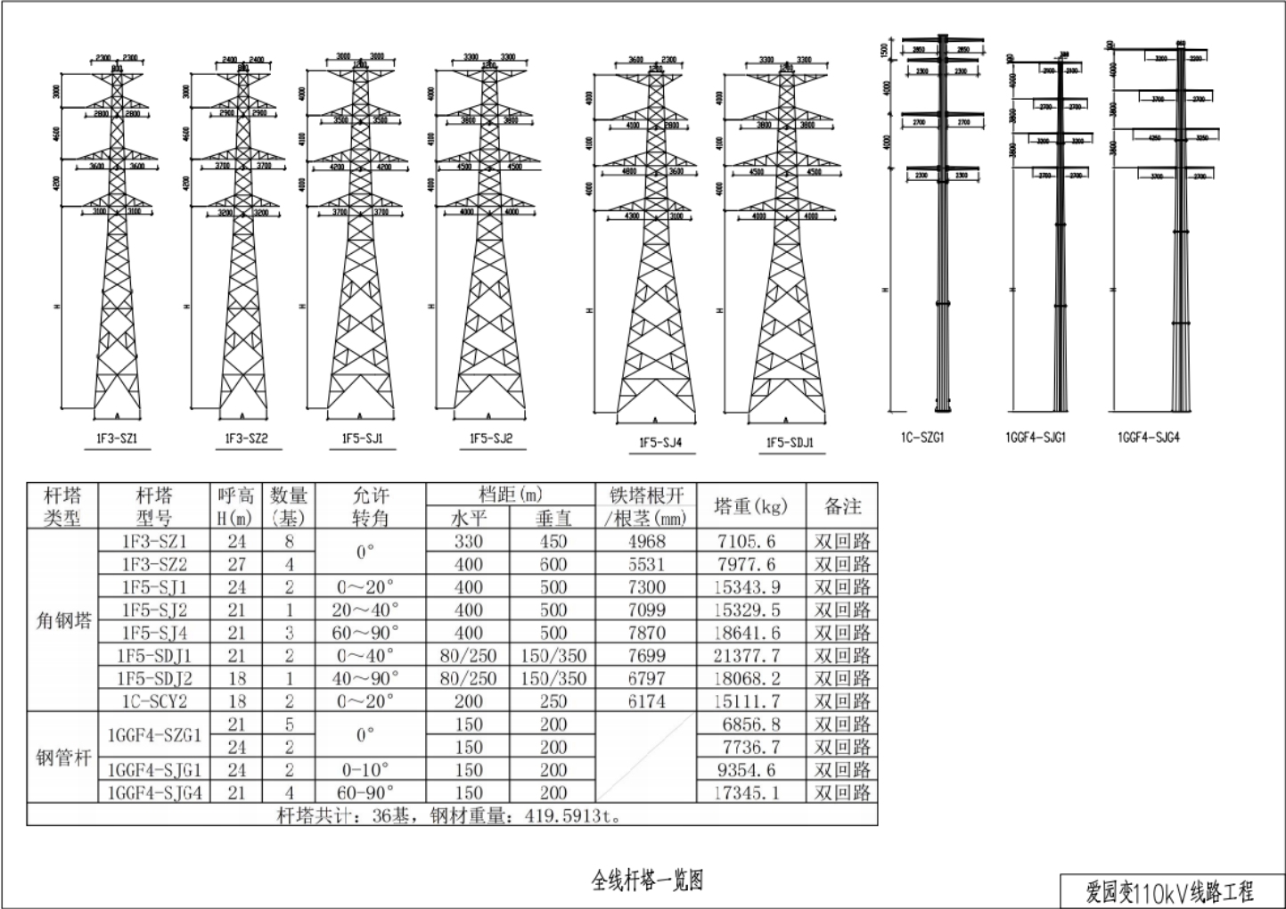
附图 6 本工程塔型图
