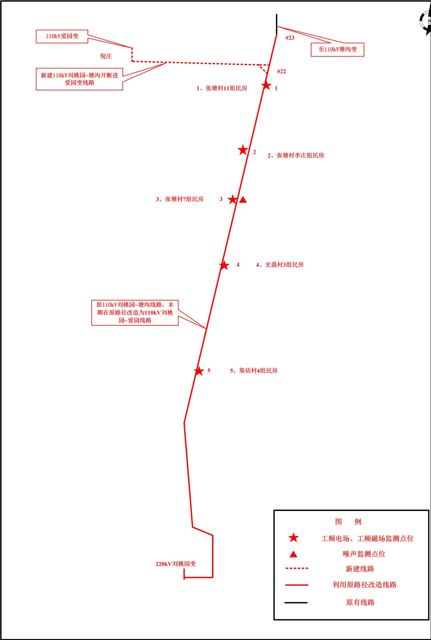
附图 4 刘桃园变至塘沟变开断环进入爱园变 110kV 线路路径及监测点位示意图
