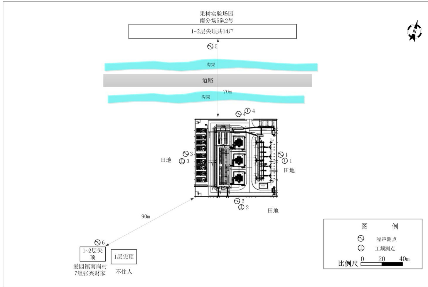
附图 2 110kV 爱园变电站拟建址周围监测点位及环境示意图
