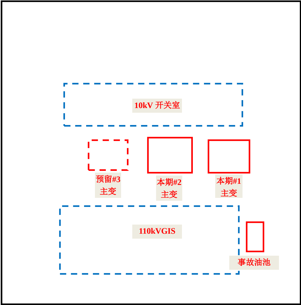
附图 3 110kV 穿城变电站总平面布置示意图
