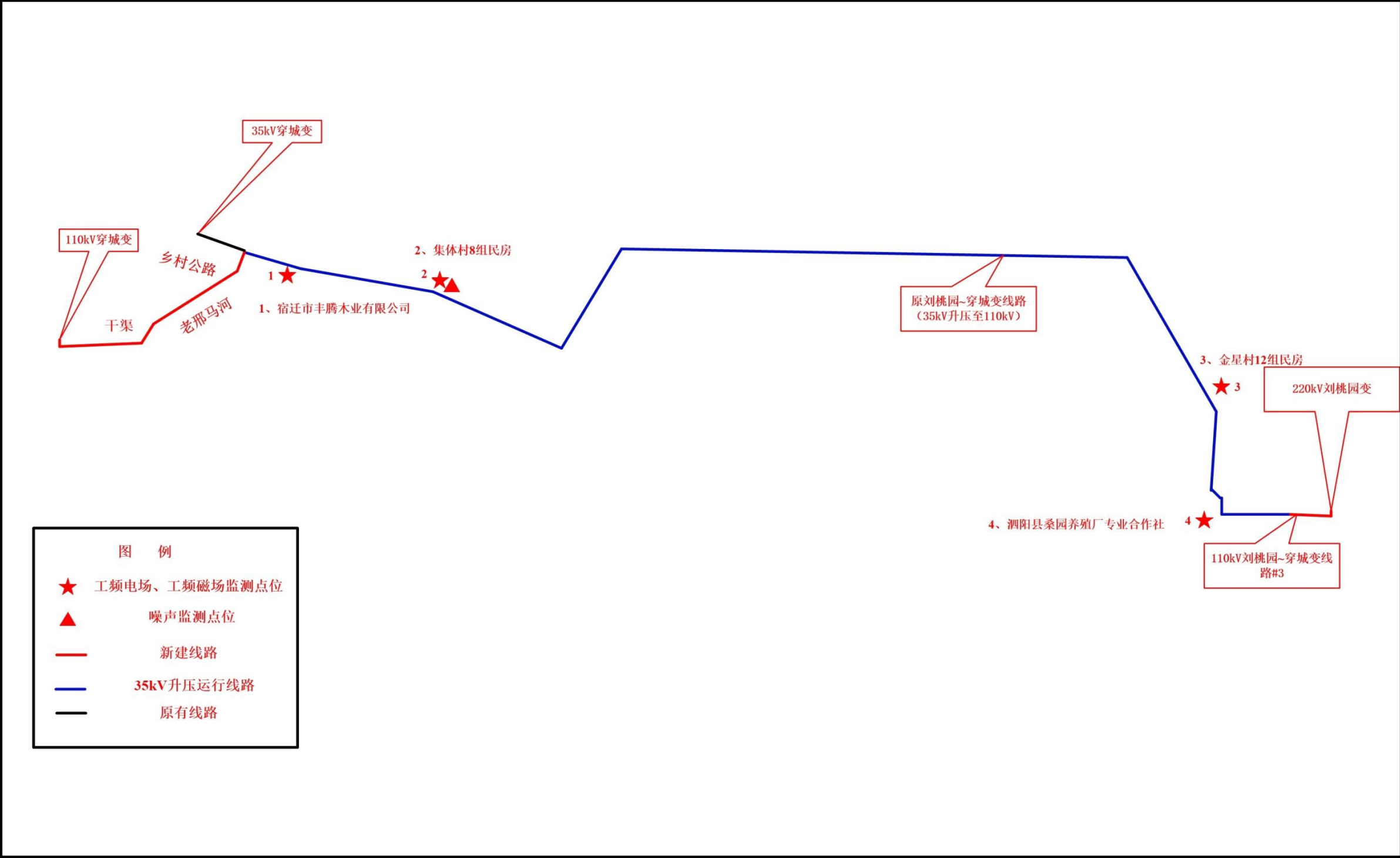
附图 4 刘桃园变至穿城变 110kV 路路径及监测点位示意图
