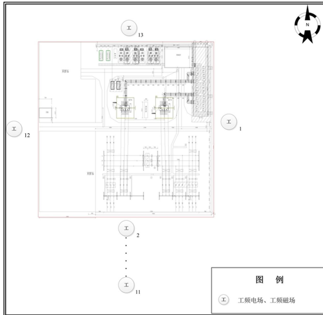
附图 6 110kV 城南变电站（类比站）监测点位示意图
