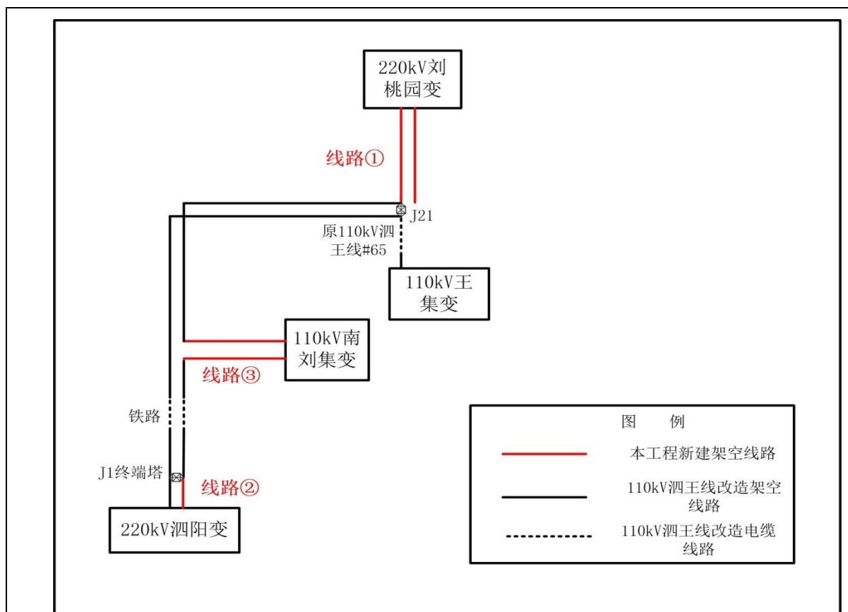
图 1 本工程接线示意图
