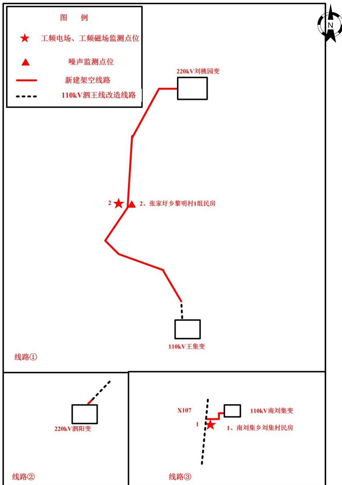
附图 4 刘桃园~泗阳开断环入南刘集变 110kV 线路路径及监测点位示意图
