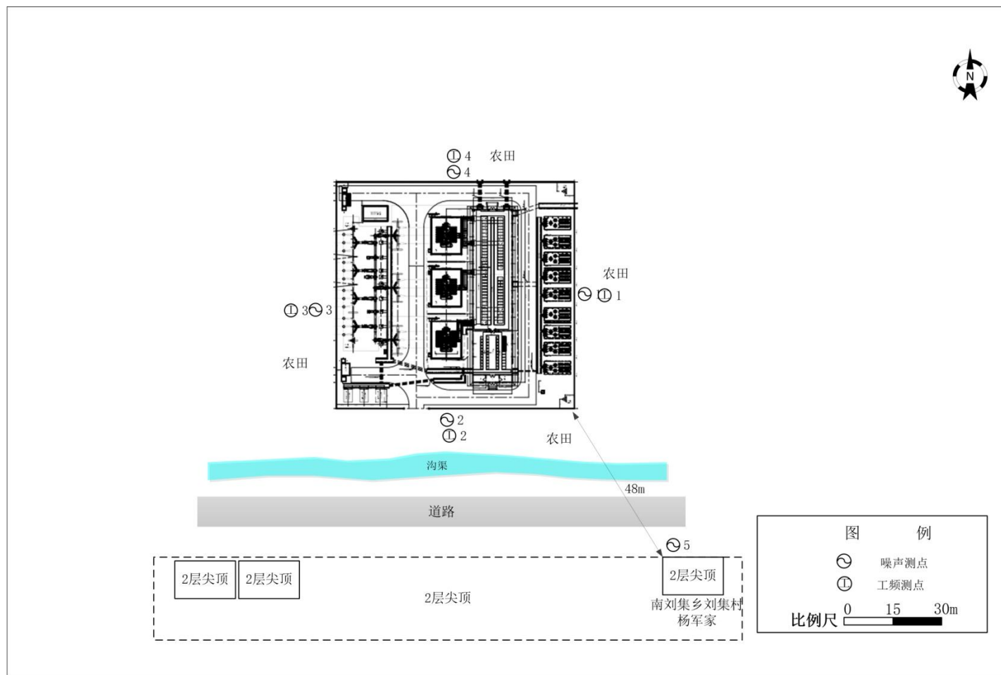
附图 2 110kV 南刘集变电站拟建址周围监测点位及环境示意图
