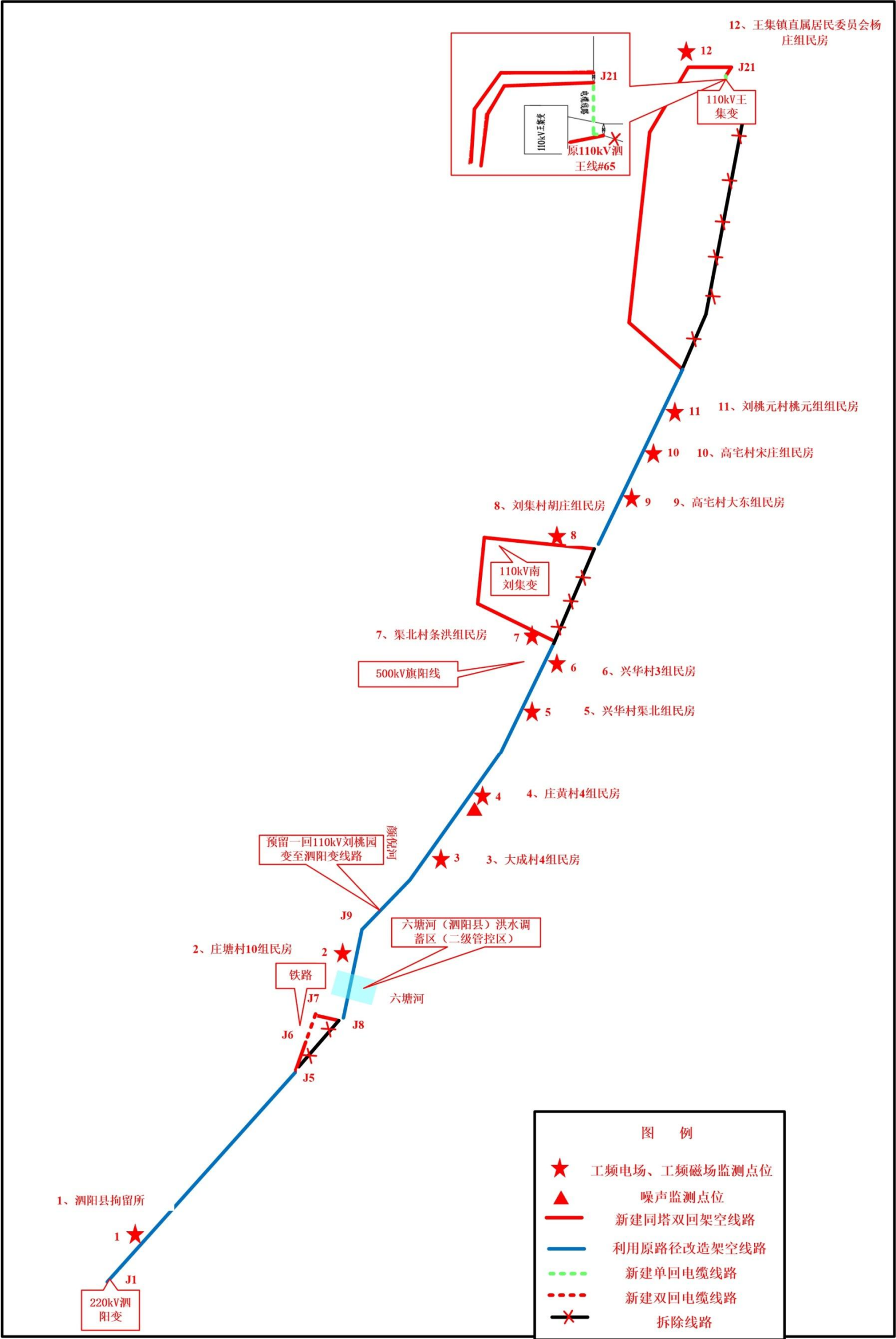
附图 2 110kV 泗王线改造工程线路路径及监测点位示意图
