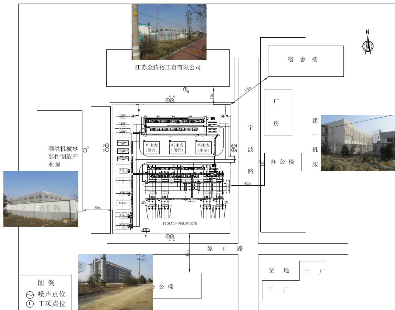
附图2 110kV 田桥变电站监测点位及周围环境示意图
