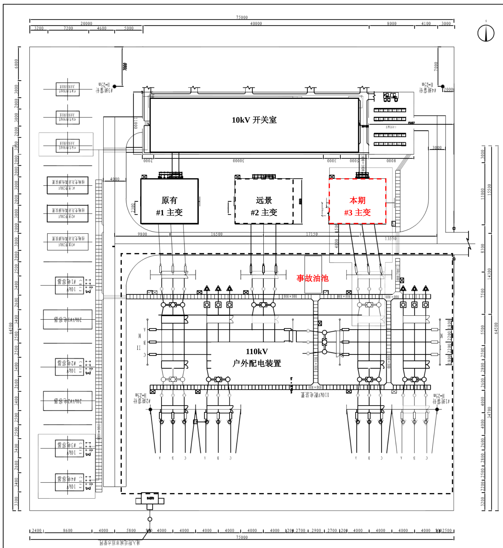
附图 3 110kV 田桥变电站平面布置示意图
