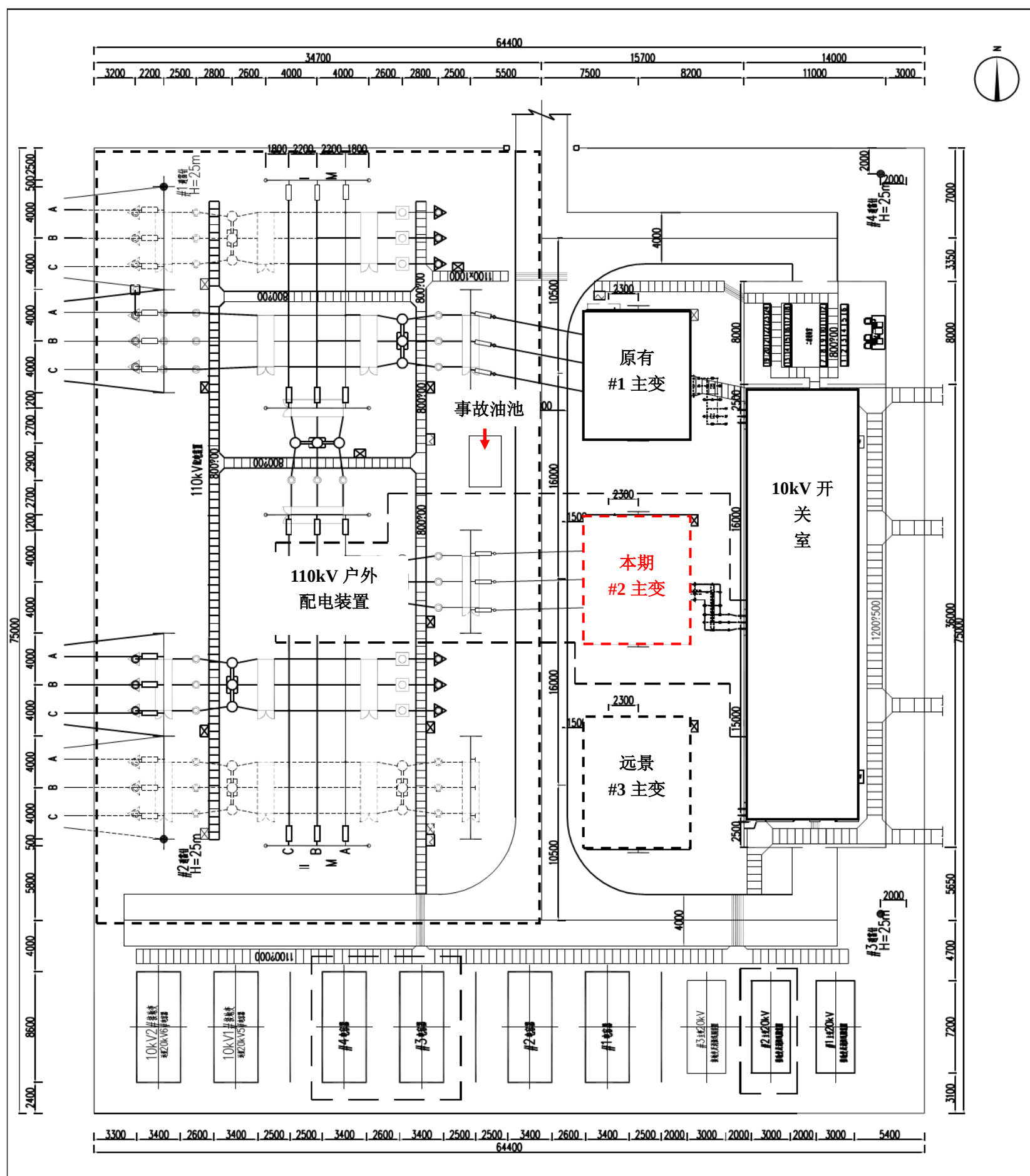
附图 3 110kV 柴米变电站平面布置示意图
