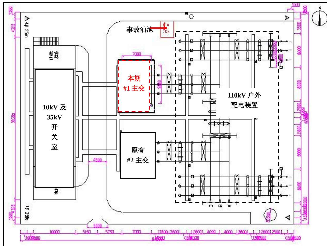
附图 3 110kV 胡集变电站平面布置示意图
