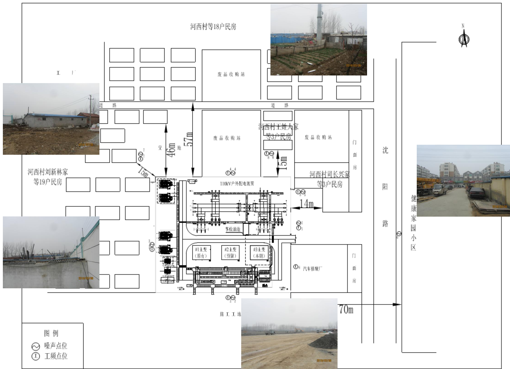
附图2 110kV南湖变电站监测点位及周围环境示意图
