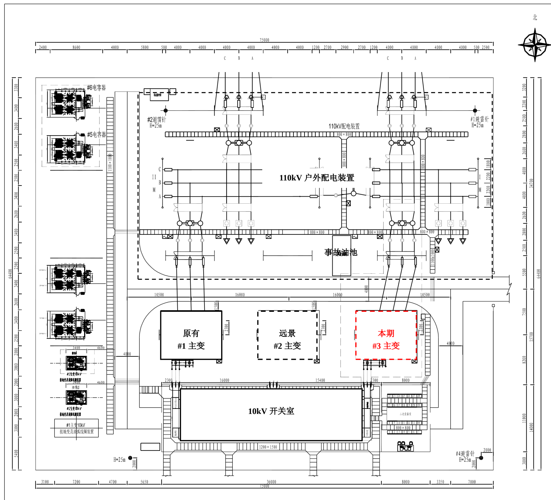
附图 3 110kV 南湖变电站平面布置示意图
