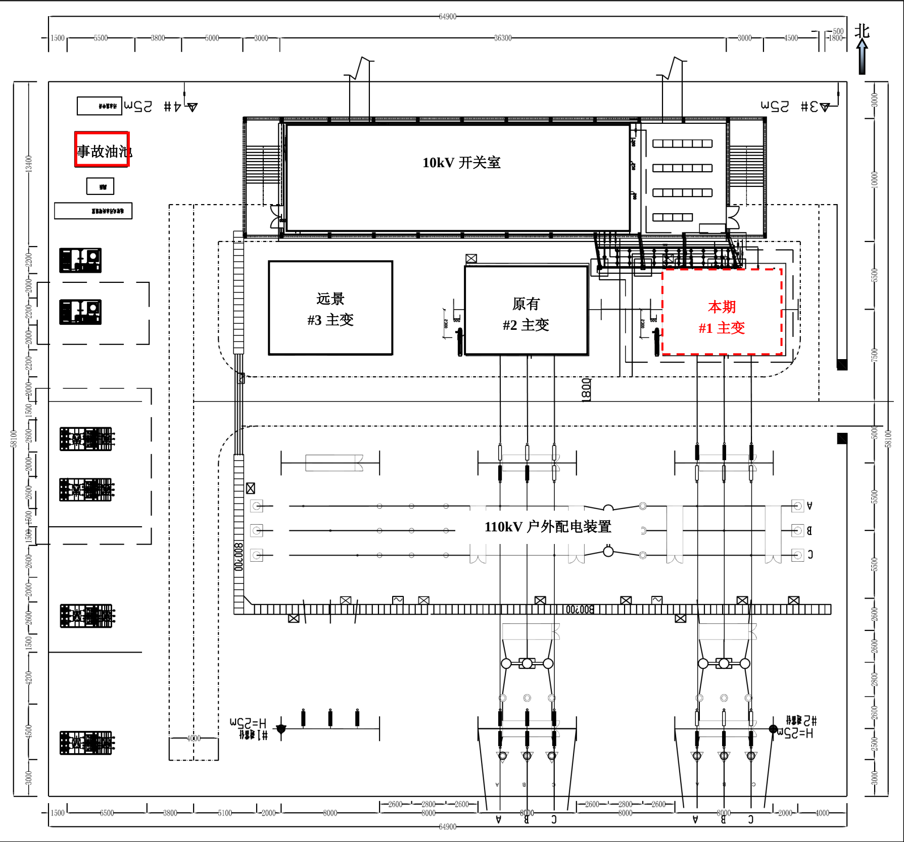
附图3 110kV扎下变电站平面布置示意图
