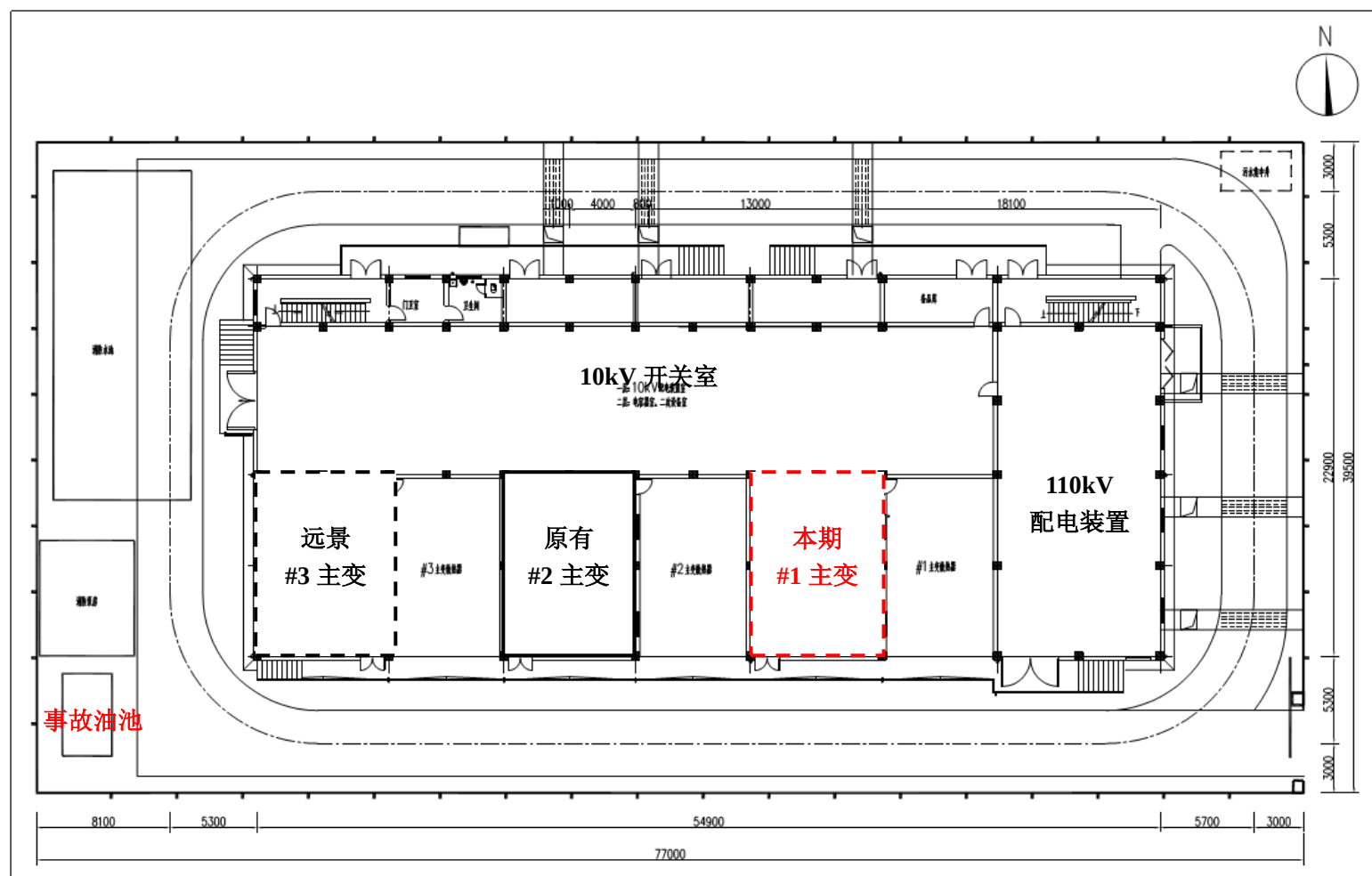
附图 3 110kV 青阳变电站平面布置示意图
