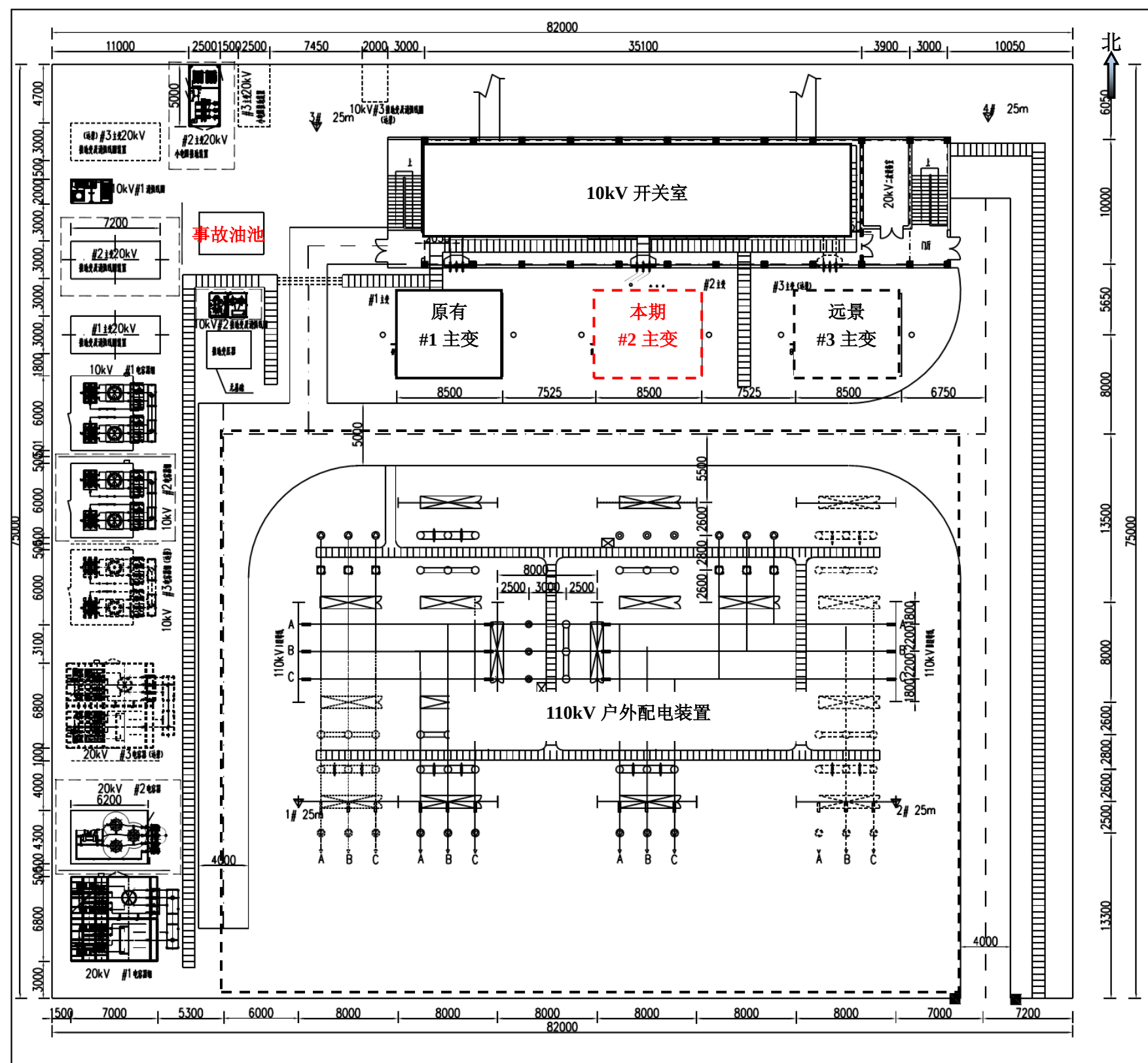
附图 3 110kV 泗洲变电站平面布置示意图
