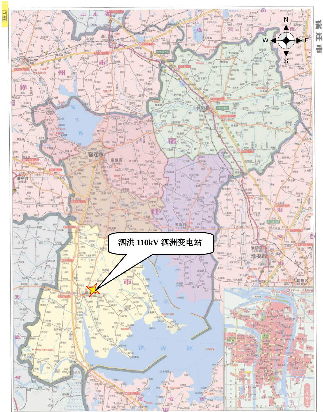
附图 1 泗洪 110kV 泗洲变电站扩建#2 主变工程地理位置示意图
