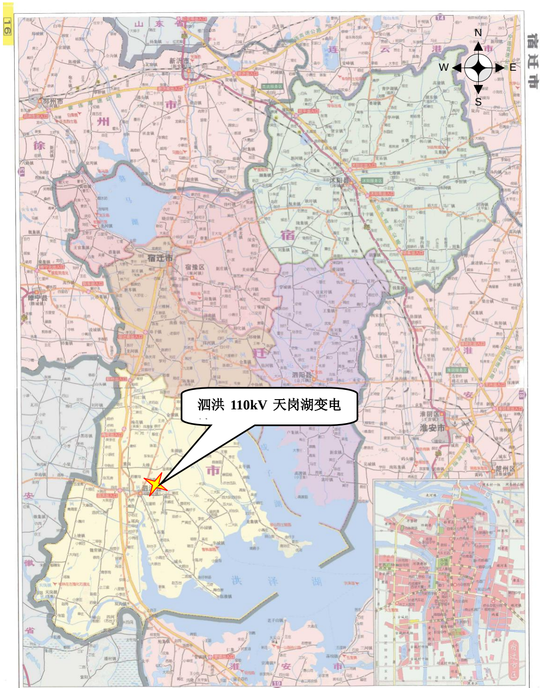
附图 1 泗洪 110kV 天岗湖变电站扩建#2 主变工程地理位置示意图
