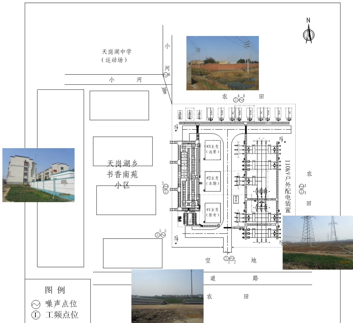
附图 2 110kV 天岗湖变电站监测点位及周围环境示意图
