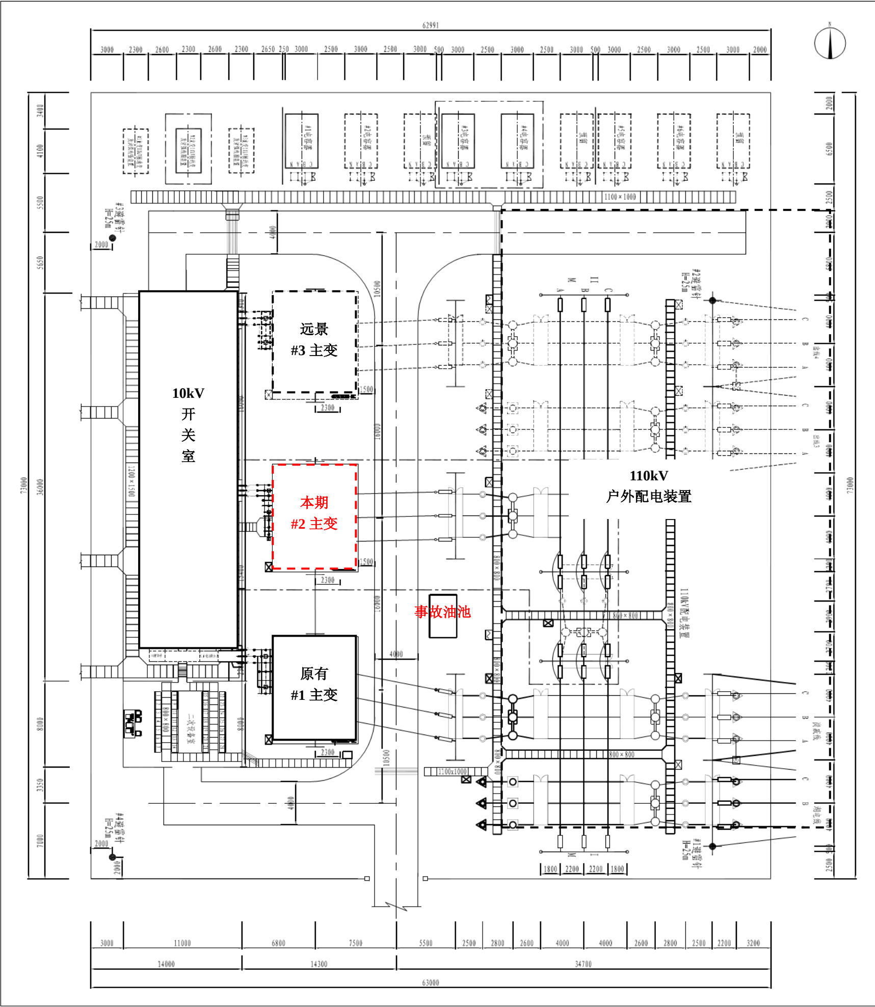
附图 3 110kV 天岗湖变电站平面布置示意图
