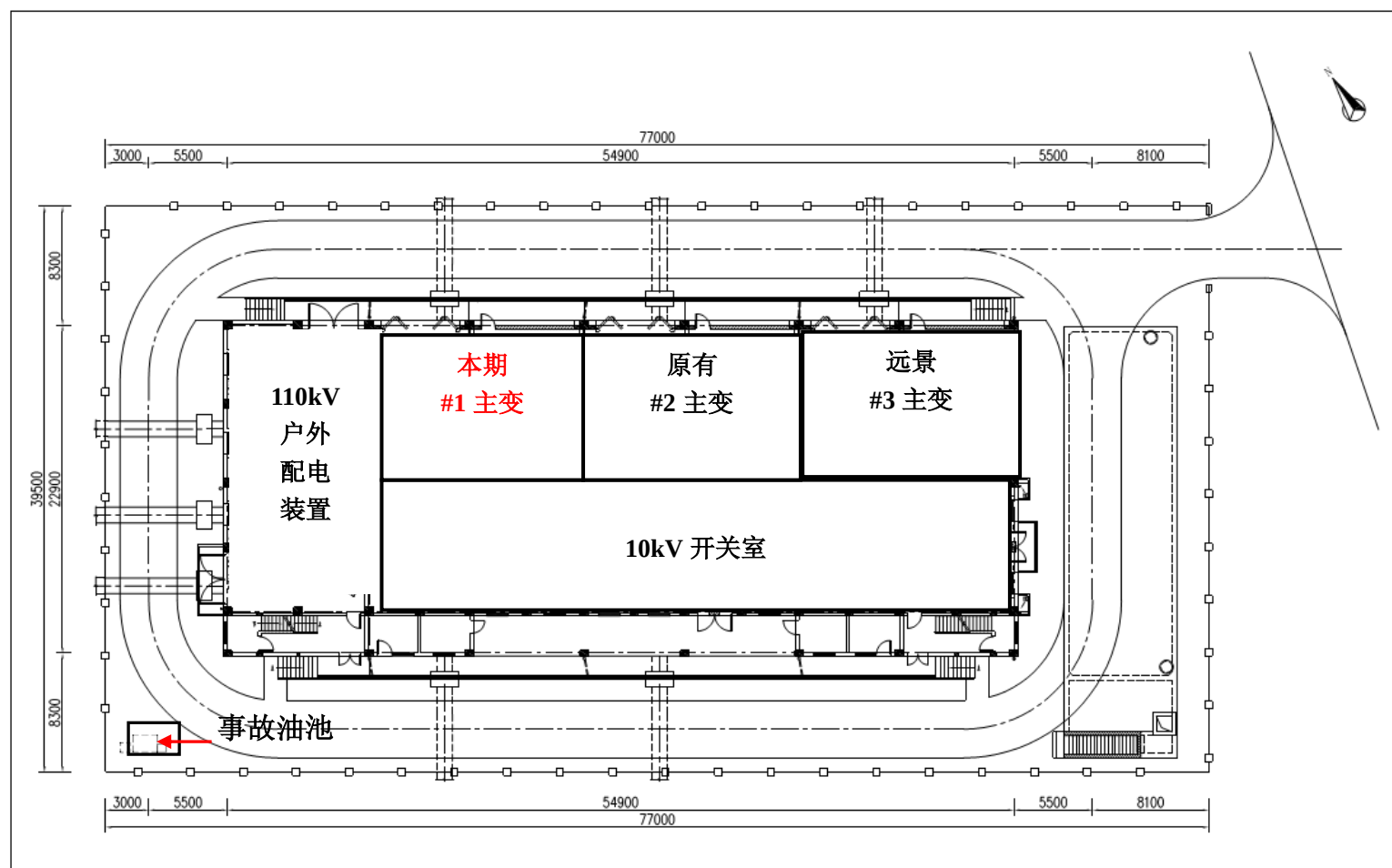
附图 3 110kV 泗水变电站平面布置示意图
