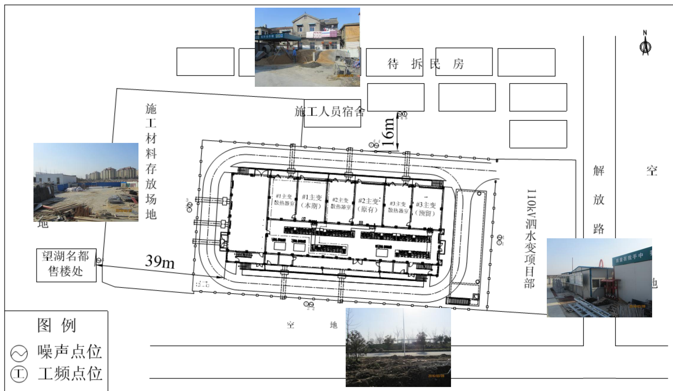
附图 2 110kV 泗水变电站监测点位及周围环境示意图
