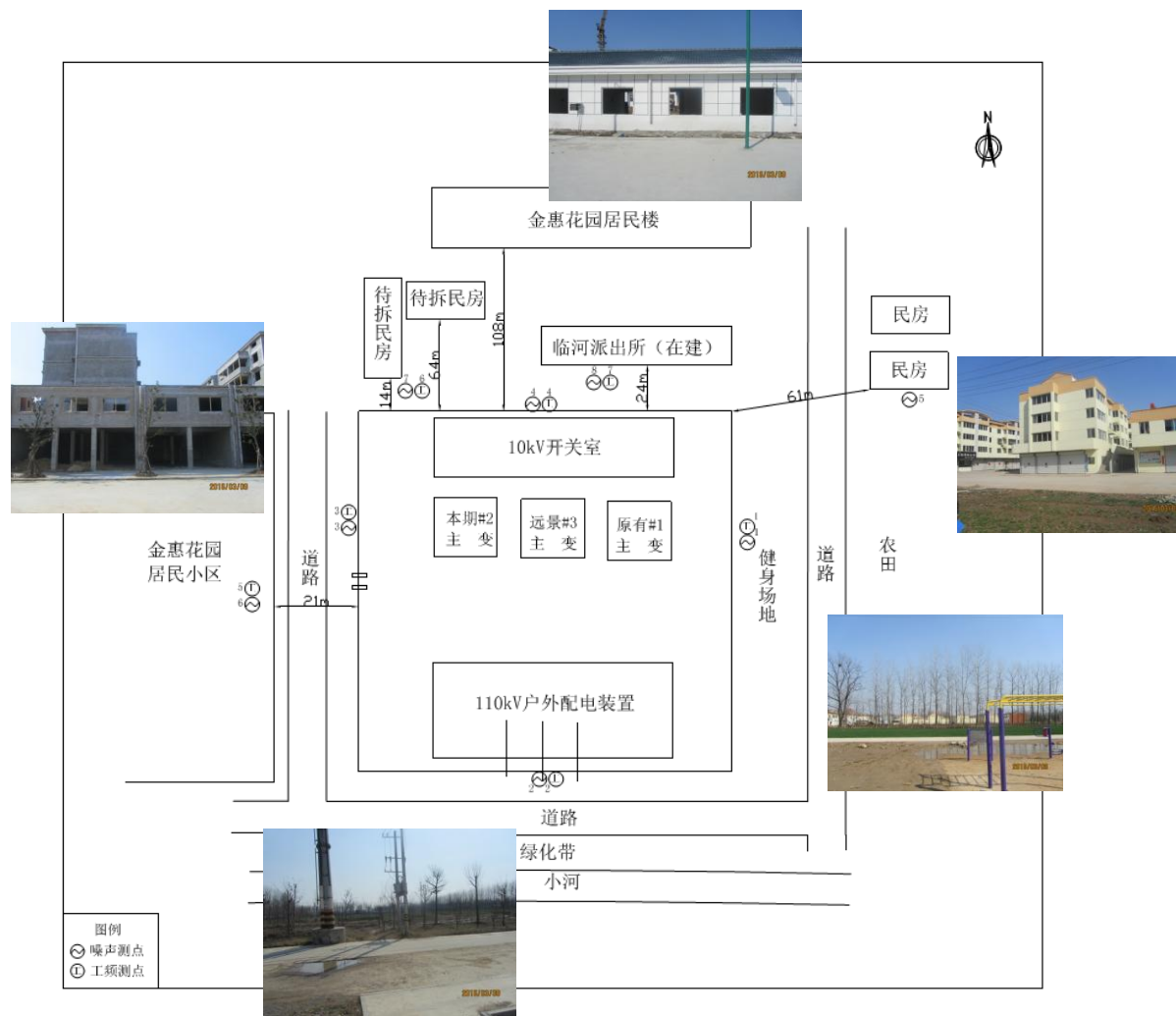
附图 2 110kV 临河变电站监测点位及周围环境示意图
