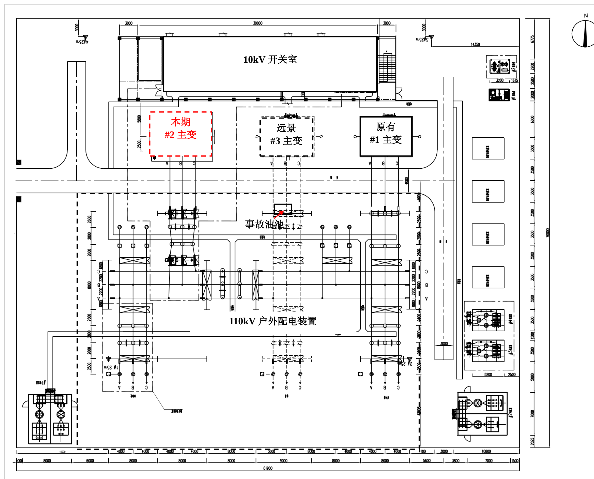
附图 3 110kV 临河变电站平面布置示意图
