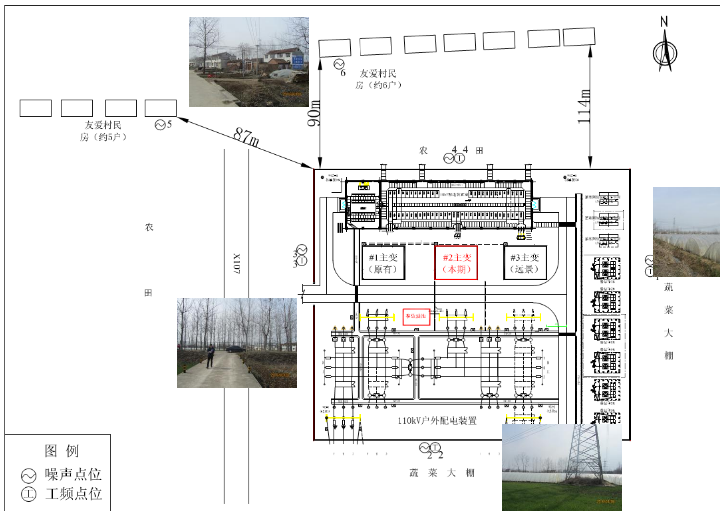
附图 2 110kV 洋北变电站监测点位及周围环境示意图
