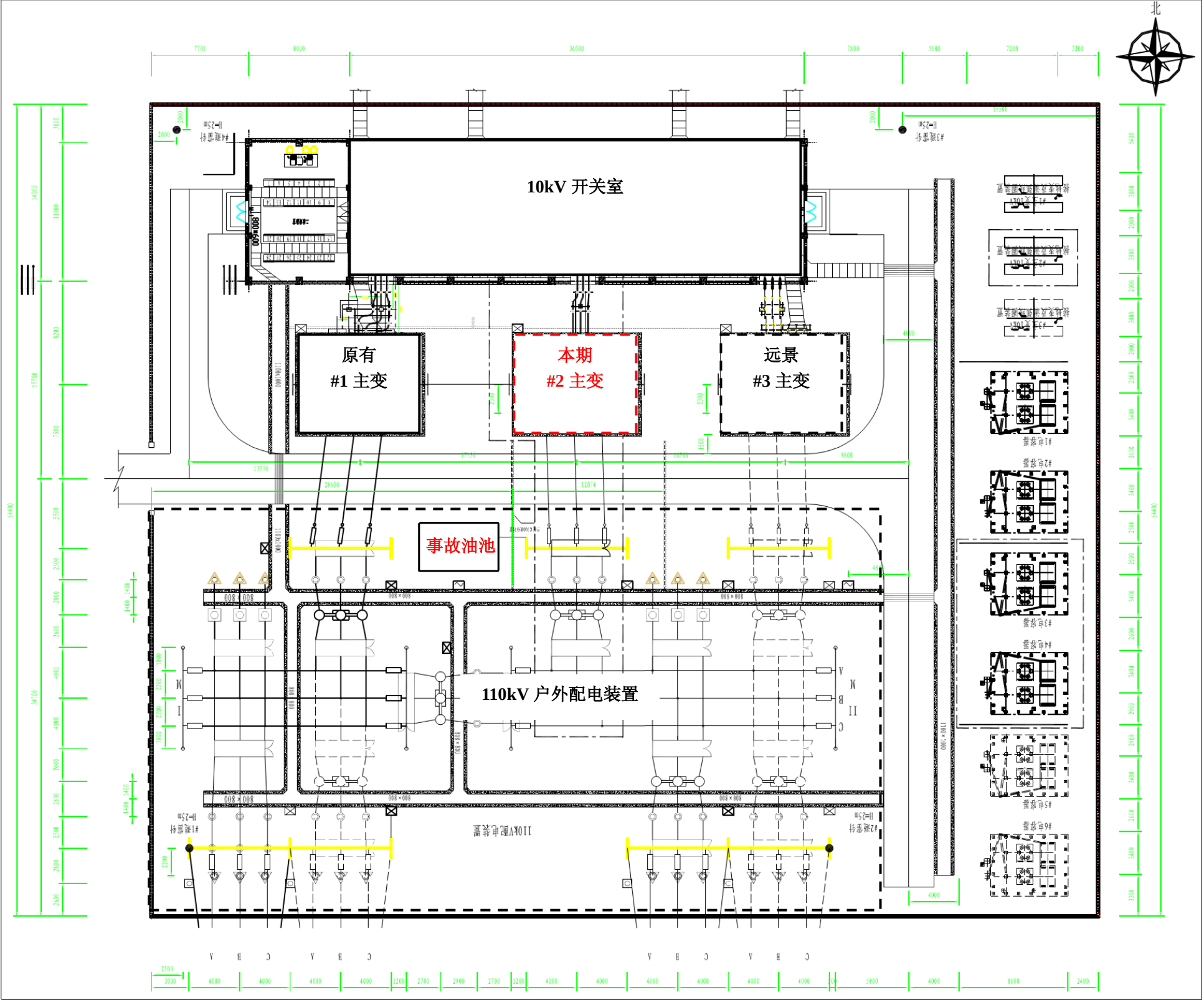
附图 3 110kV 洋北变电站平面布置示意图
