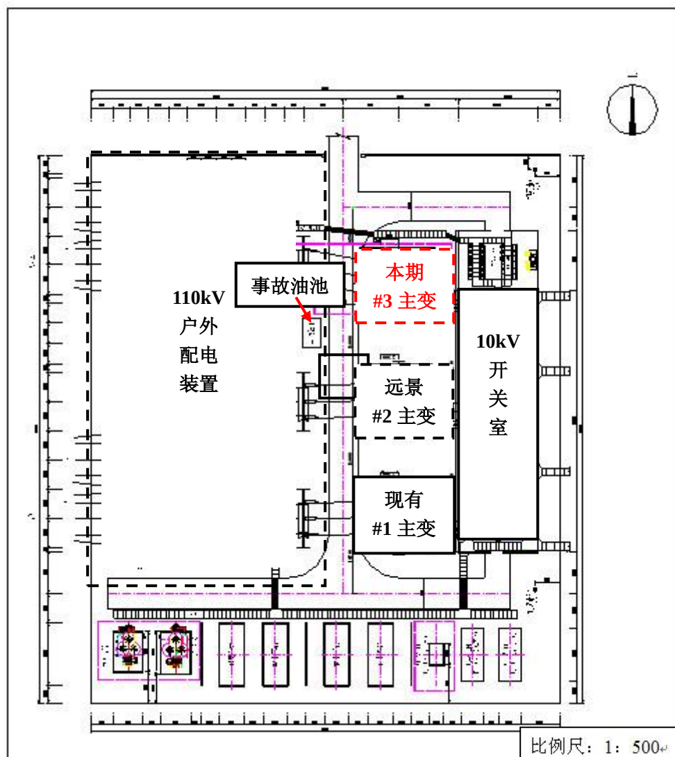
附图3 110kV 关庙变电站平面布置示意图
