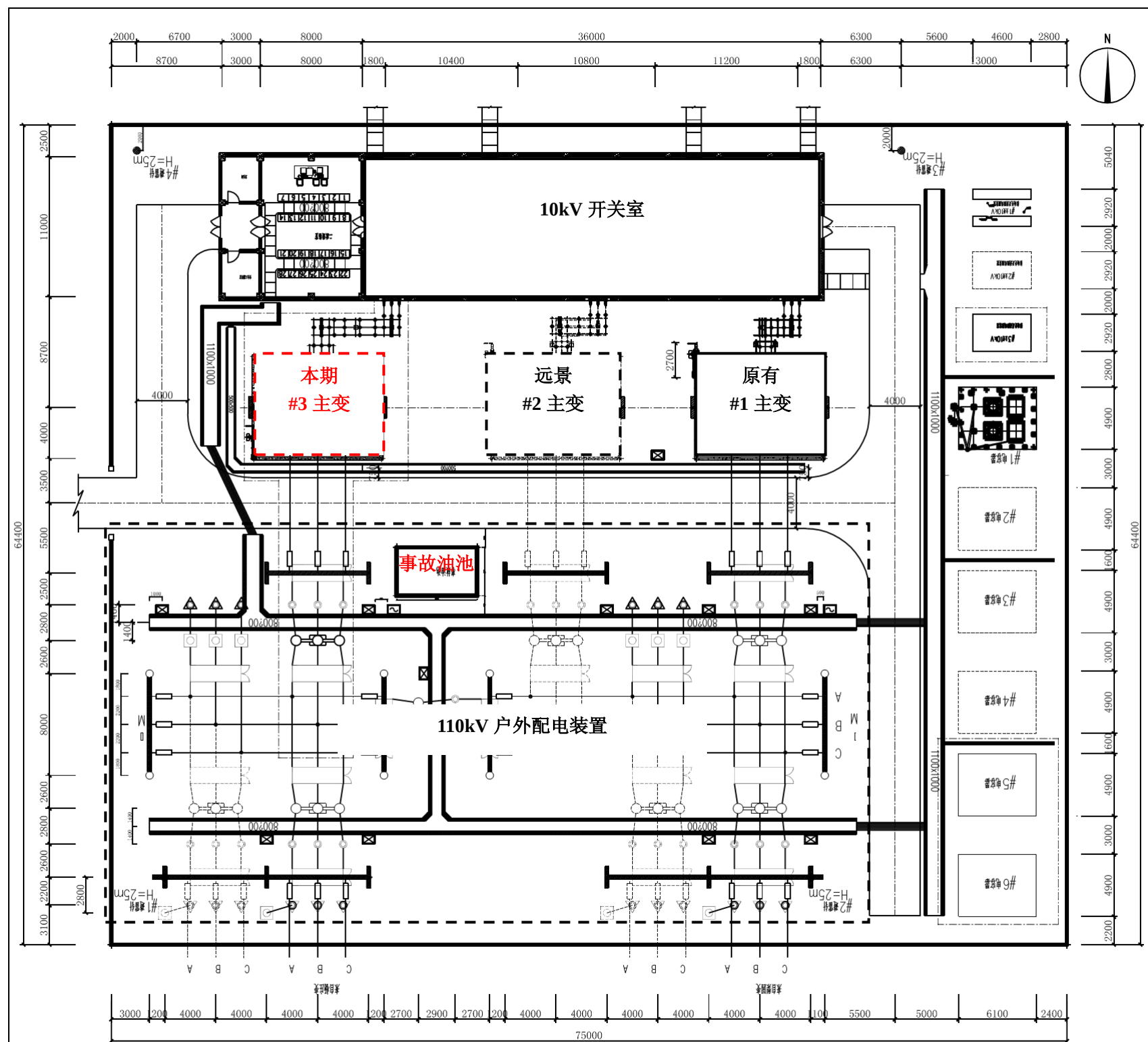
附图 3 110kV 龙河变电站平面布置示意图
