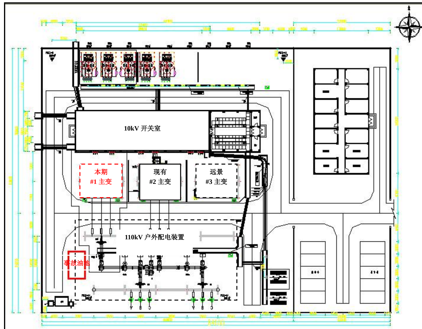
附图 3 110kV 钱塘变电站平面布置示意图
