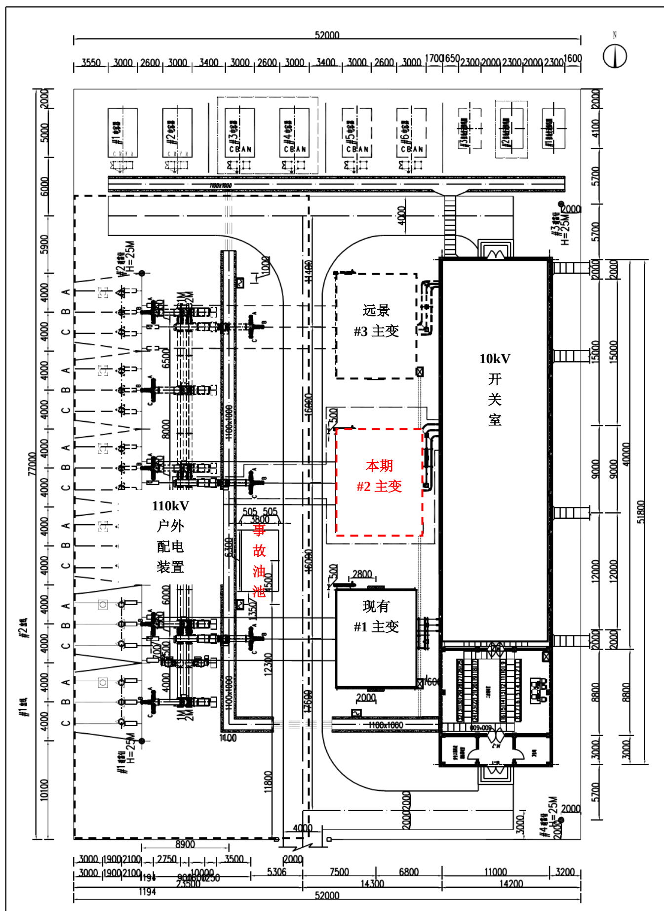
附图 2 110kV 通湖变电站平面布置图
