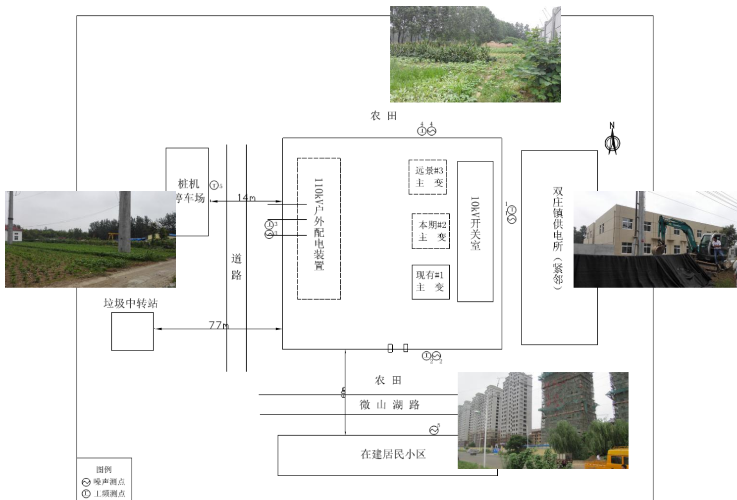
附图 2 110kV 通湖变电站监测点位及周围环境示意图
