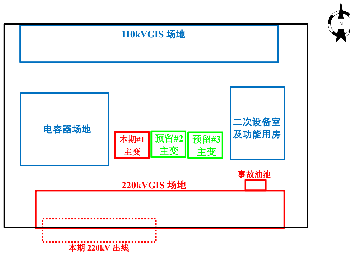
附图 3 220kV 周巷变电站平面布置示意图
