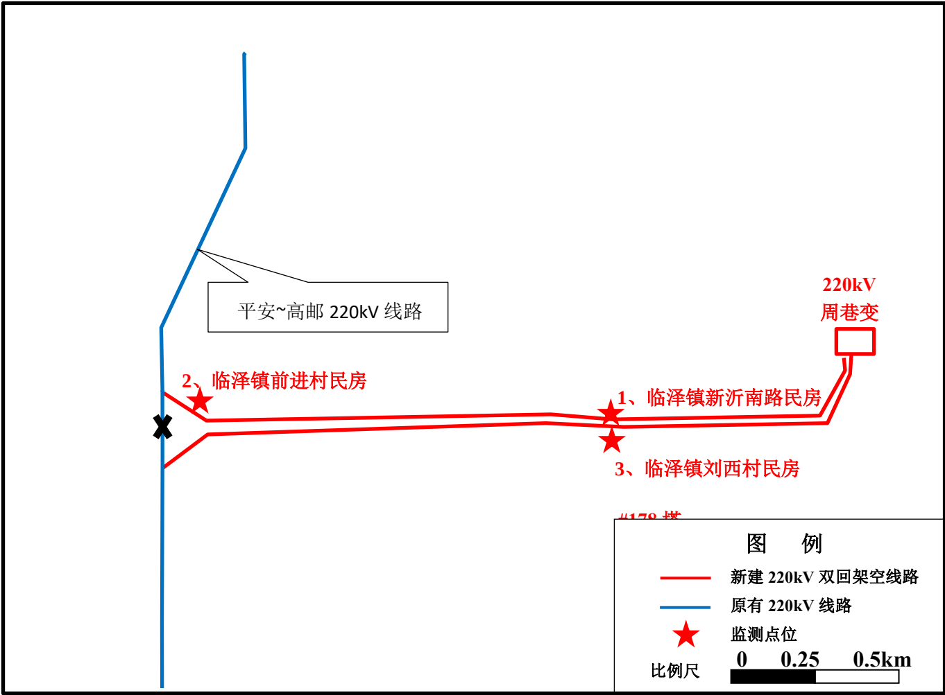
附图 4 220kV 周巷变配套线路路径及监测点位示意图
