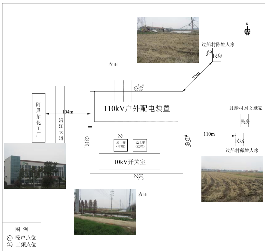
附图2 110kV 过船变电站监测点位及周围环境示意图
