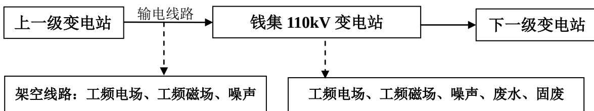
图 1 宿迁钱集 110kV 输变电工程工艺流程及产污环节示意图
