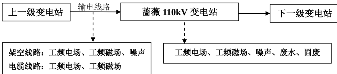
图 1 宿迁蔷薇 110kV 输变电工程工艺流程及产污环节示意图
