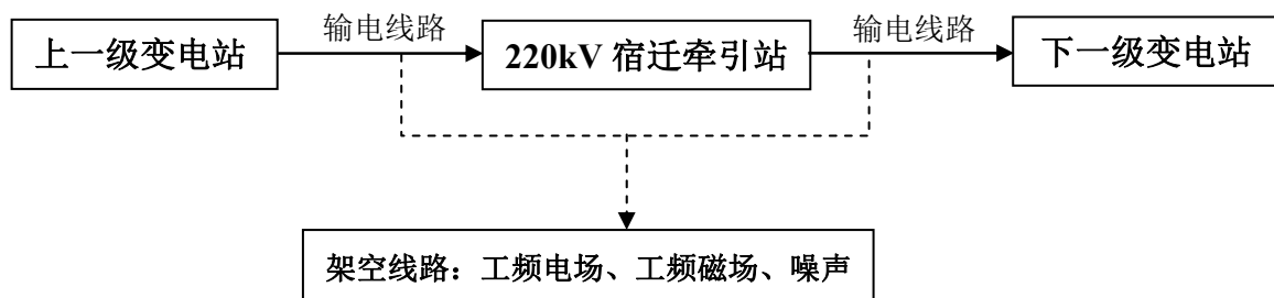
图 2 本工程工艺流程及产污环节示意图
