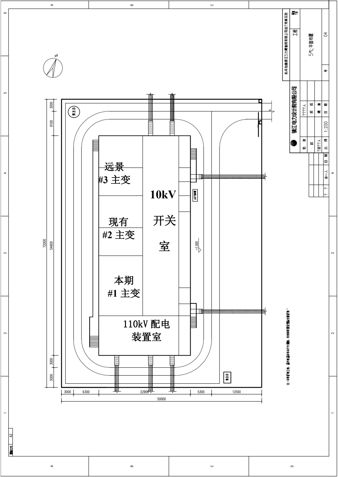
附图 4 110kV 郭庄变电站平面布置示意图
