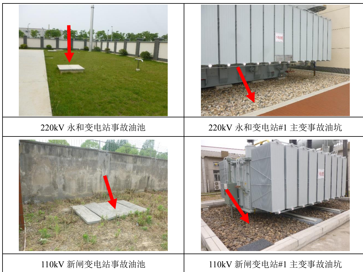
图 6-2 本批验收的变电站事故油池及事故油坑示例
