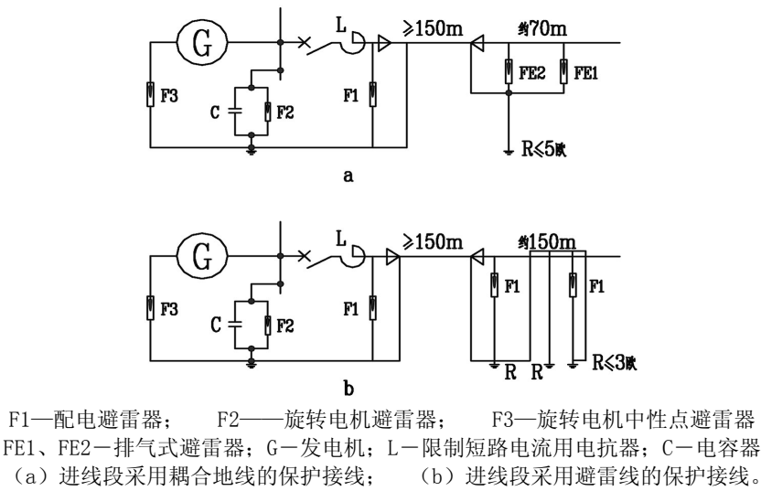
图 21 25000kW~60000kW 直配电机的保护接线
