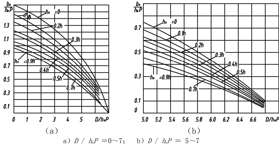
图 6 两等高 ( h ) 避雷针间保护范围的一侧最小宽度 ( b_x ) 与 D / h_P 的关系
