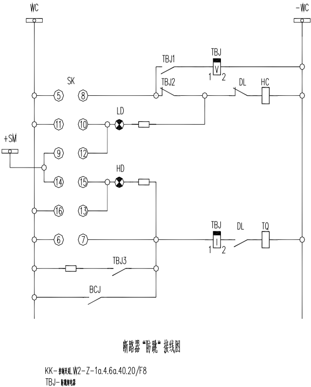
图 13.12.1 断路器“防跳”接线图
