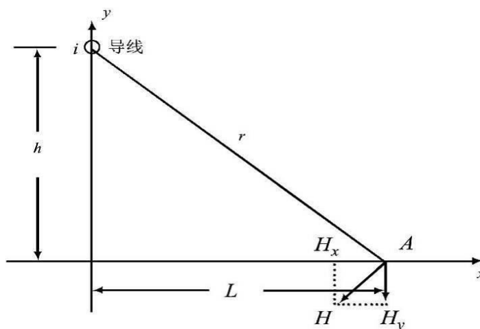
图 3.3-4 磁场向量图
