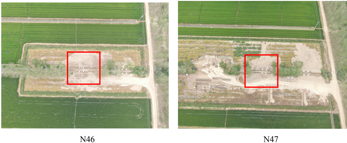
图 3-1 塔基区扰动面积现状图
