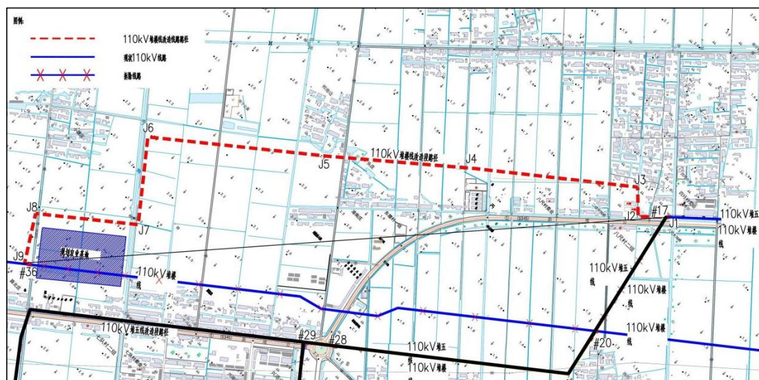
图1-1 线路路径图
