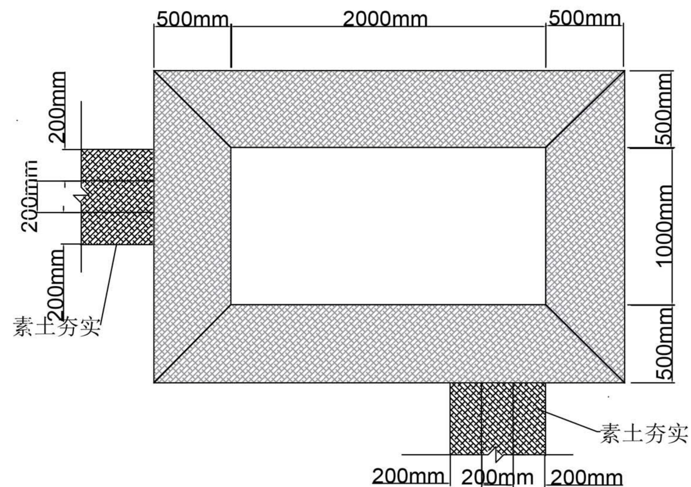
土质沉沙池（接土质排水沟）俯视图
