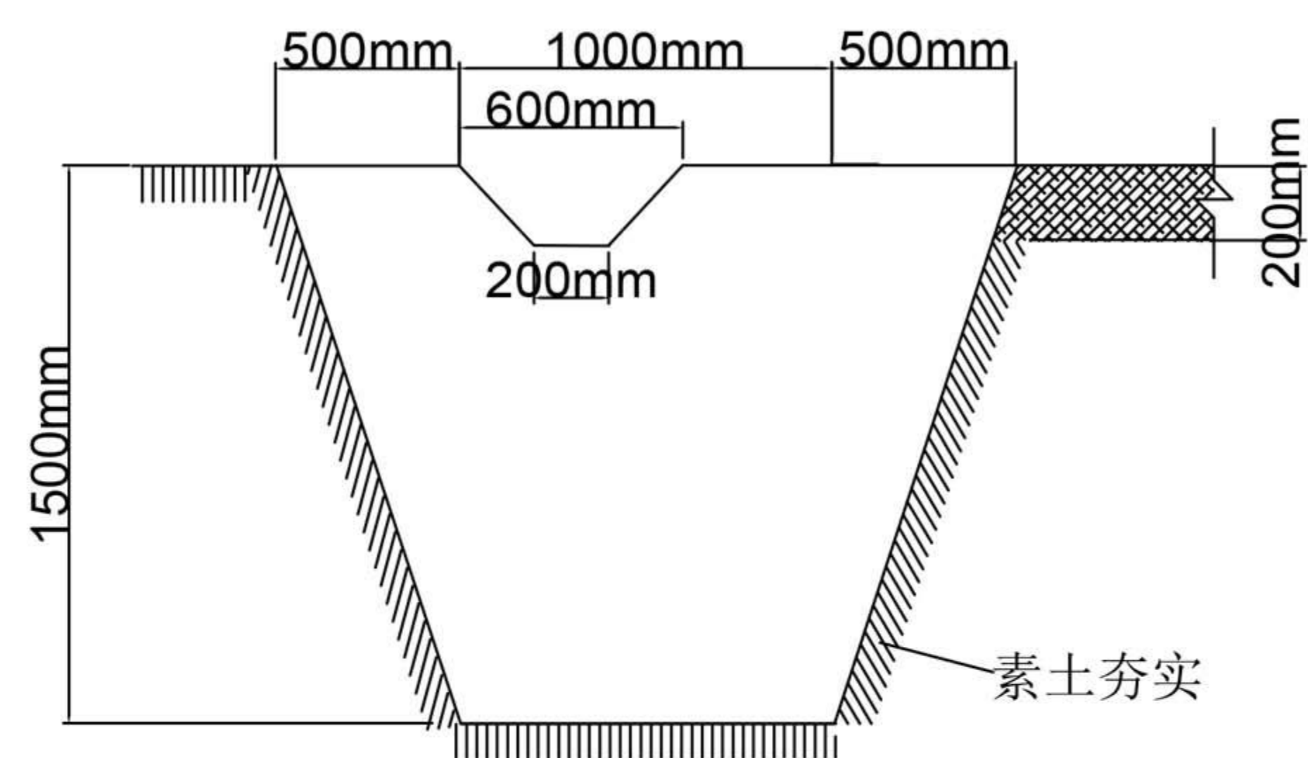
土质沉沙池（接土质排水沟）侧视图
