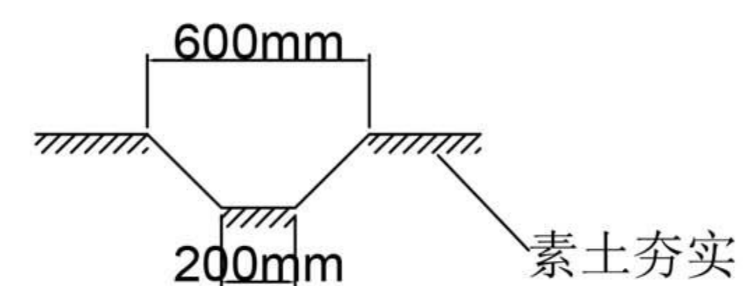
土质排水沟典型设计图
