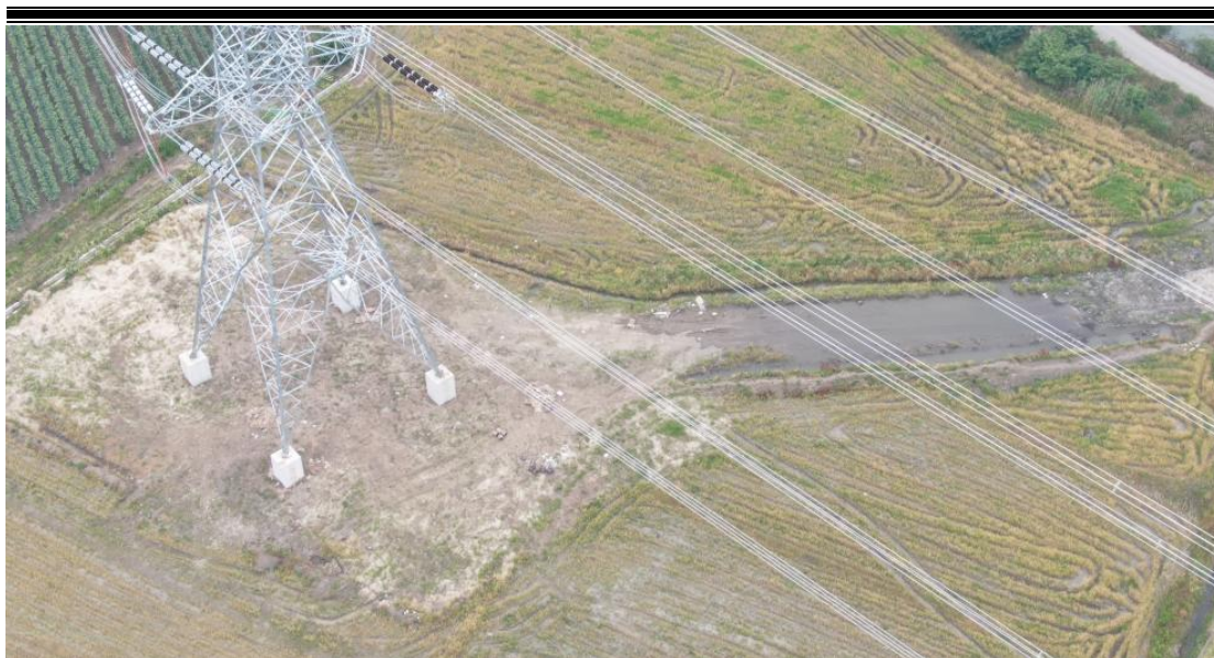
塔基及塔基施工区扰动面积图-5月
