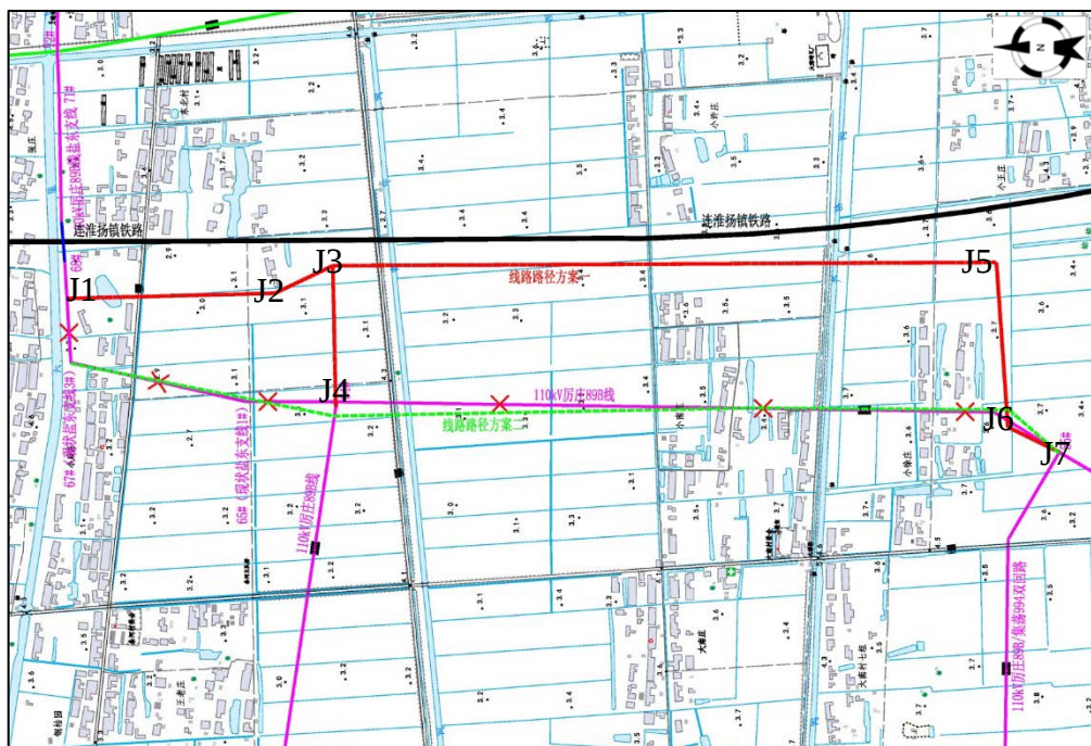
图1.1-1 线路路径图
