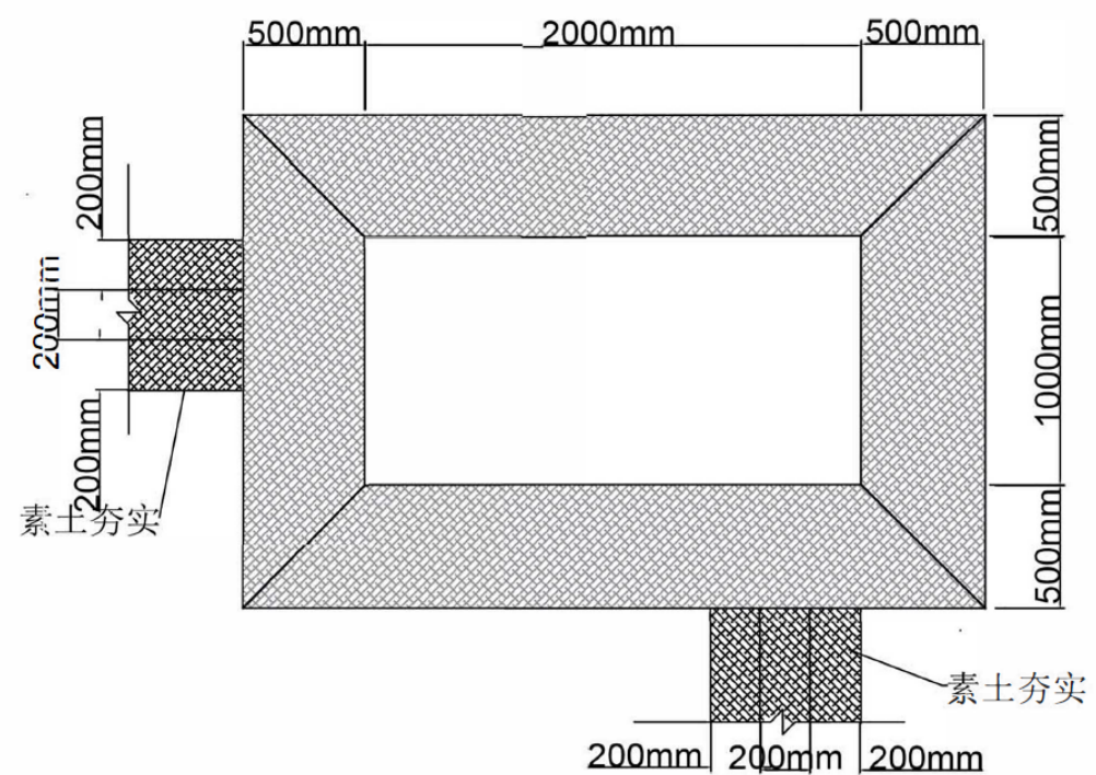
土质沉沙池（接土质排水沟）俯视图
