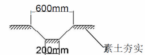
土质排水沟典型设计图
