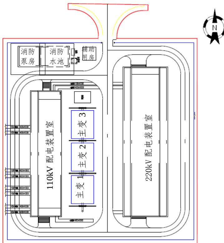
图 1 220kV 双庙变平面布置图
