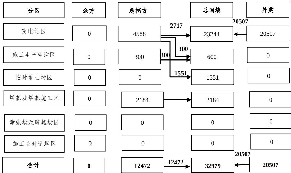
图 1-4 土石方平衡流向框图 单位: m³
