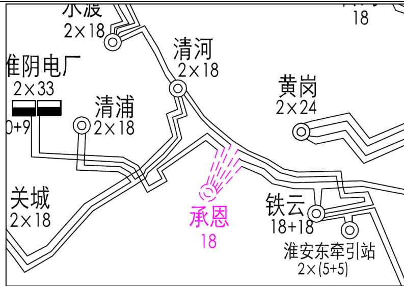
图 2-1 本项目接线示意图
