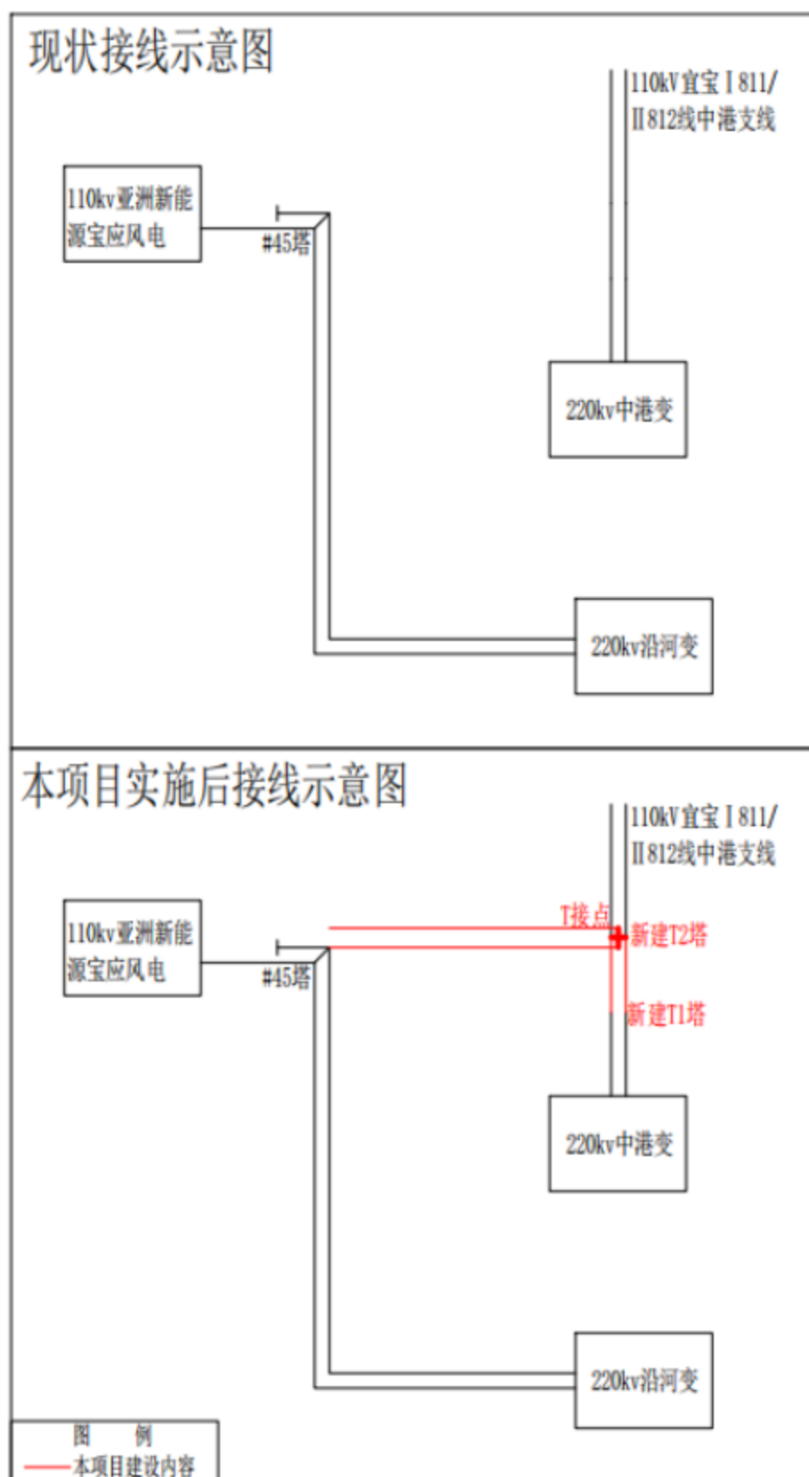
图 2-1 接线示意图
