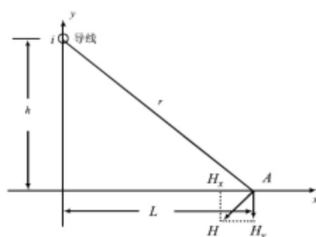
图 3.1-4 磁场向量图
