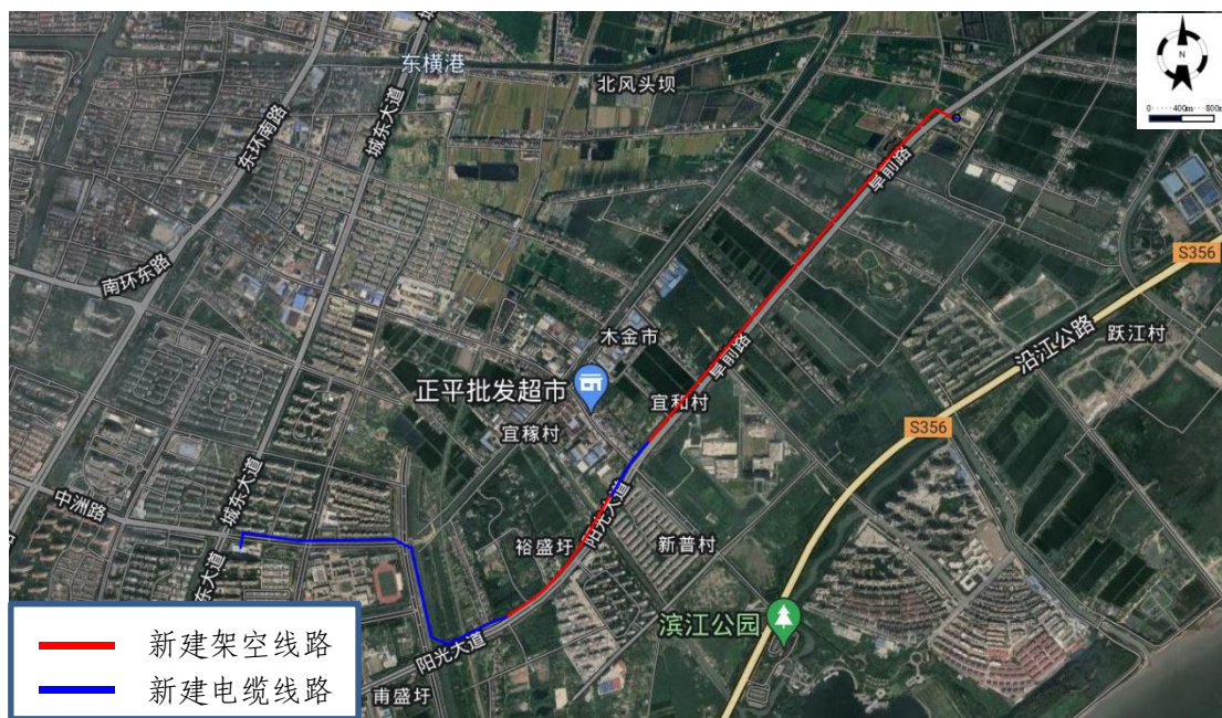
图 1.1-1 本工程线路路径走向图
