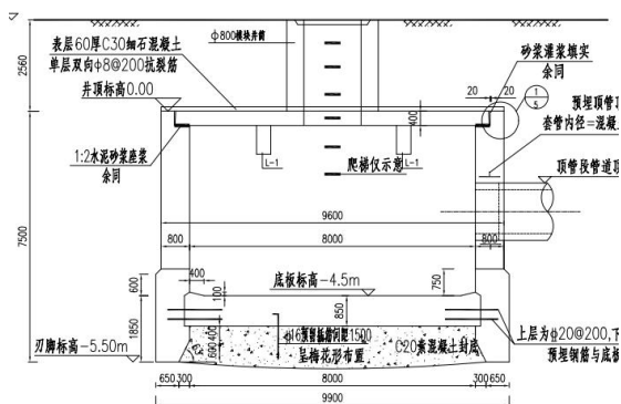
图 1.1-9 电缆工作井土建断面图
