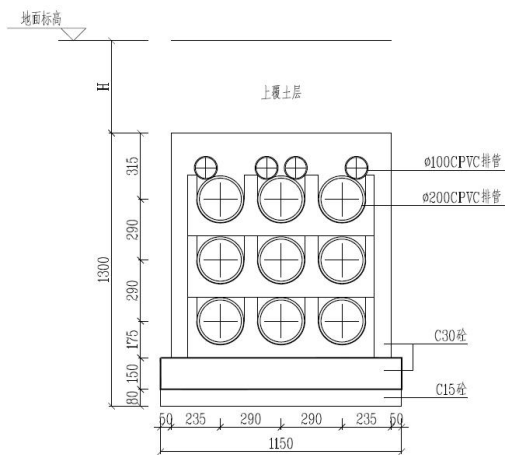
图 1.1-7 电缆排管土建断面图
