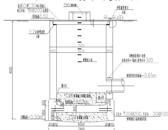
图 1.1-10 电缆接收井土建断面图
