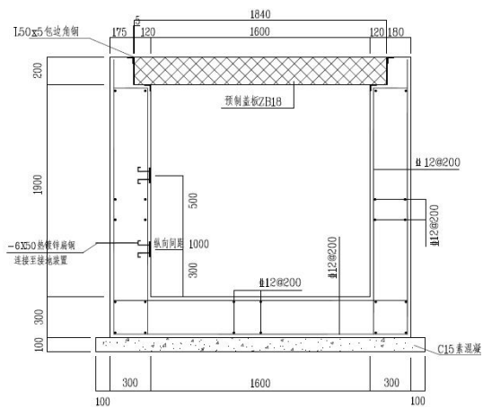
图 1.1-8 电缆沟土建断面图
