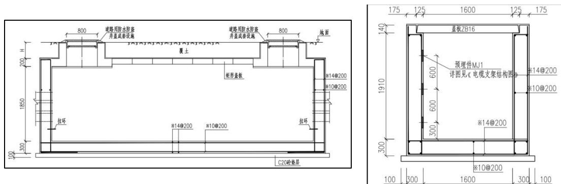
图 1.1-6 电缆井土建断面图
