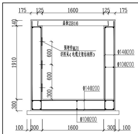
图 1.1-6 电缆沟断面图
