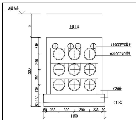
图 1.1-5 排管断面图
