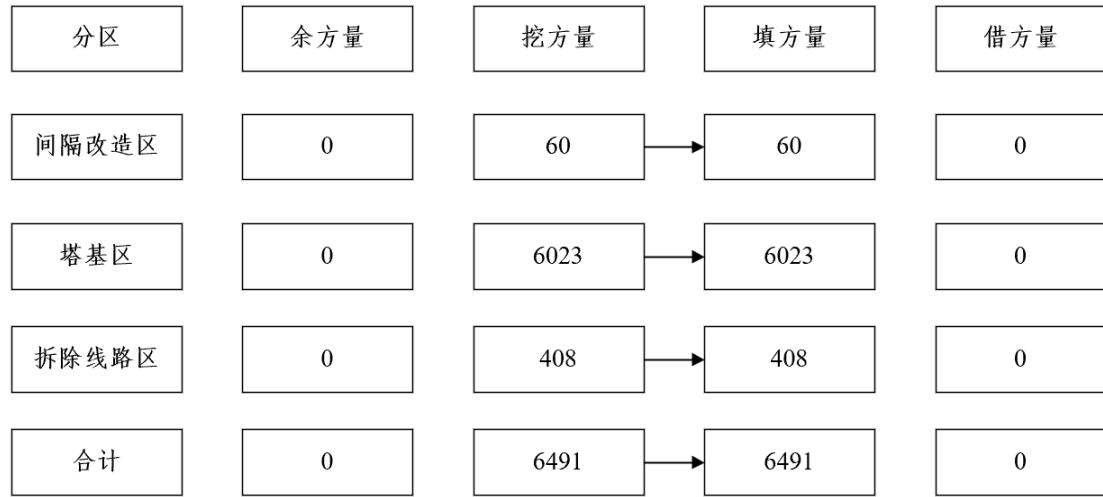
图 1.1-3 土石方平衡流向框图 单位: m 3
