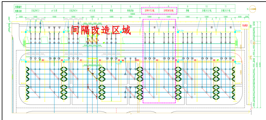
图 1.1-1 五洲 220 千伏变电站 220kV 间隔改造工程总平面布置图
