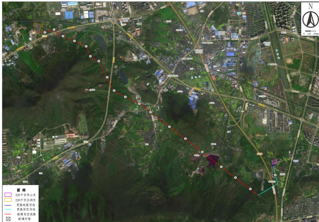
图 1.1-2 工程线路路径图
