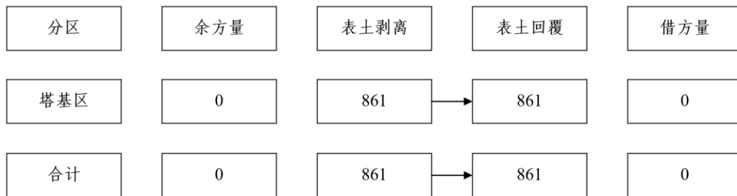
图 1.1-4 表土平衡流向框图 单位: m 3
